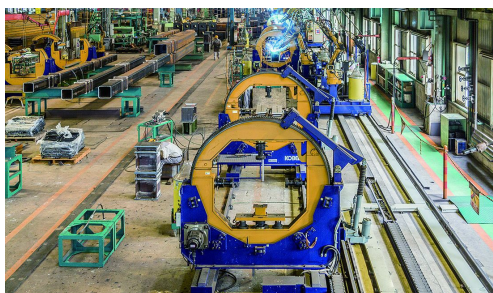
自動溶接機(柱ライン)
