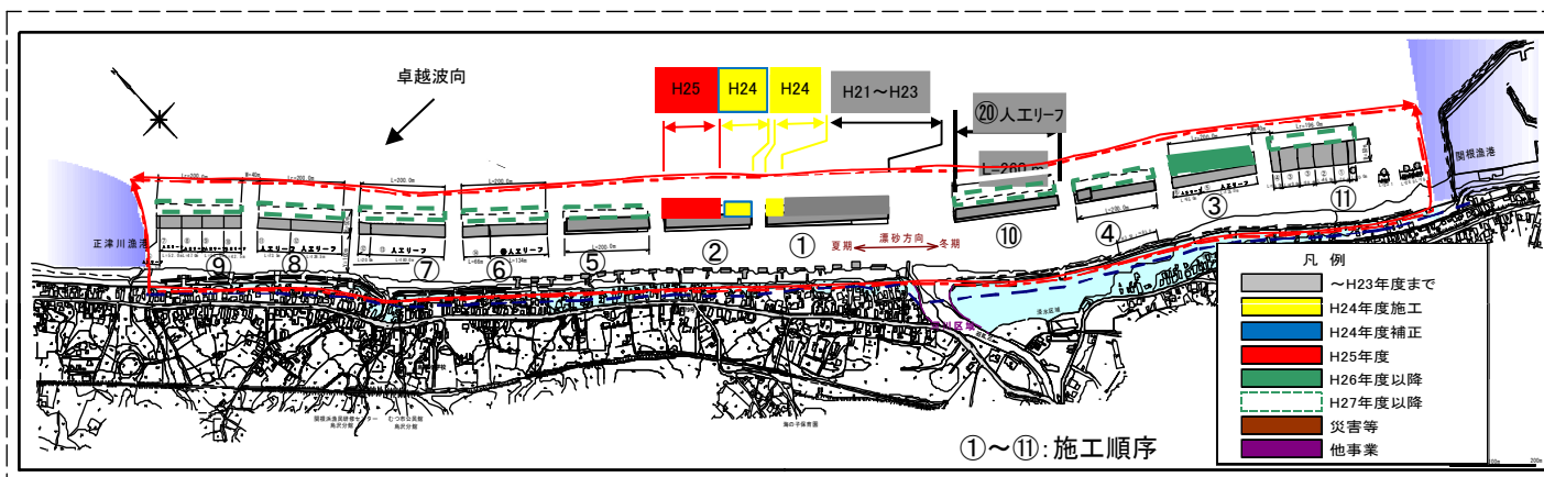
(2) 全体計画平面図
