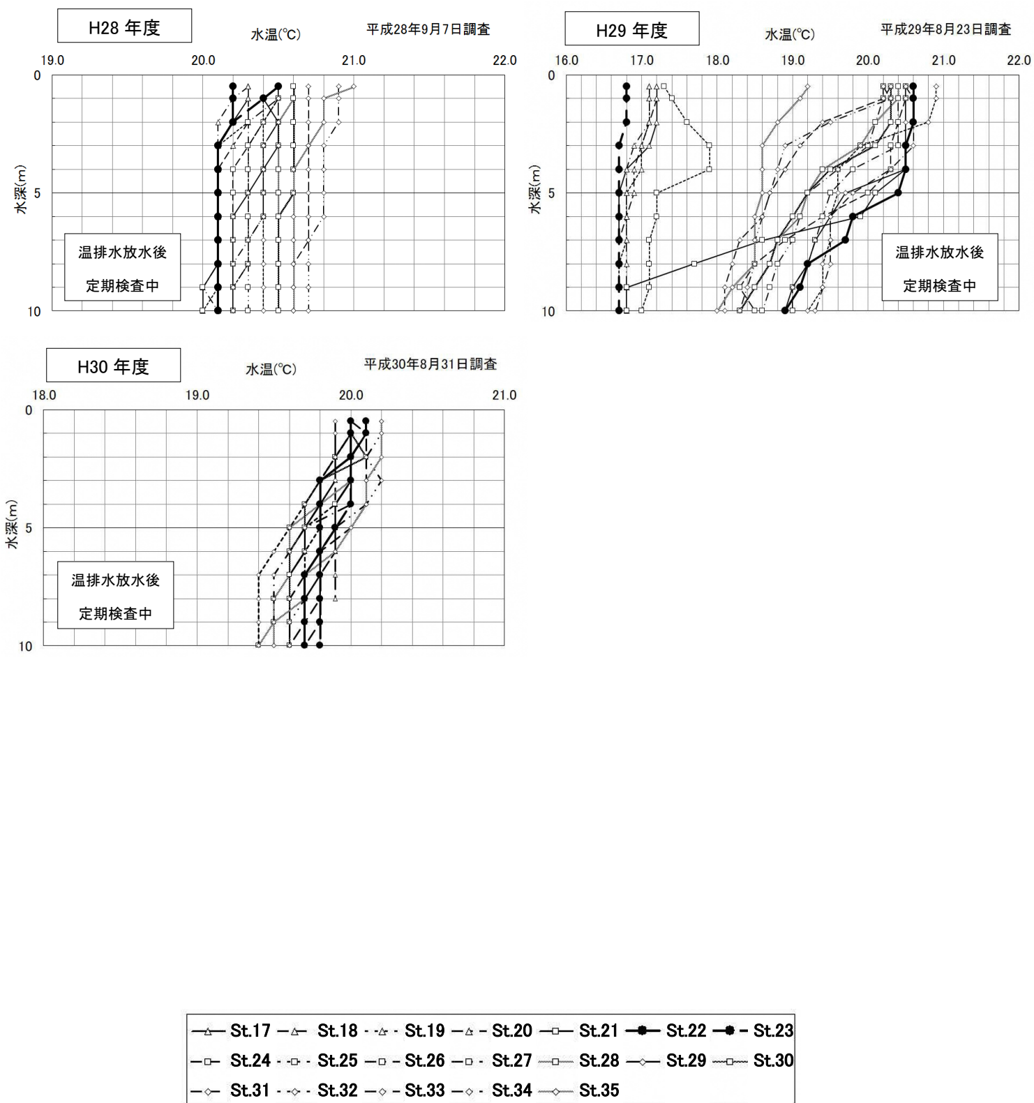
図一3.2(3) 第2四半期水温鉛直分布
