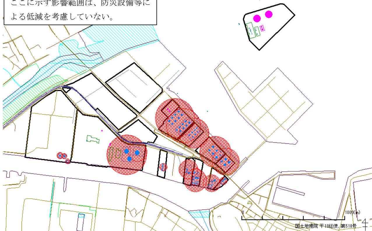
図 4.3.1 八戸地区 危険物タンクの防油堤全面火災
