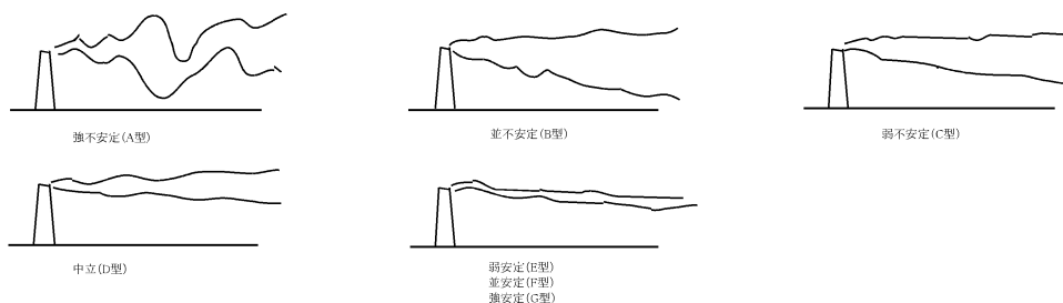
大気安定度と操の型との模式
