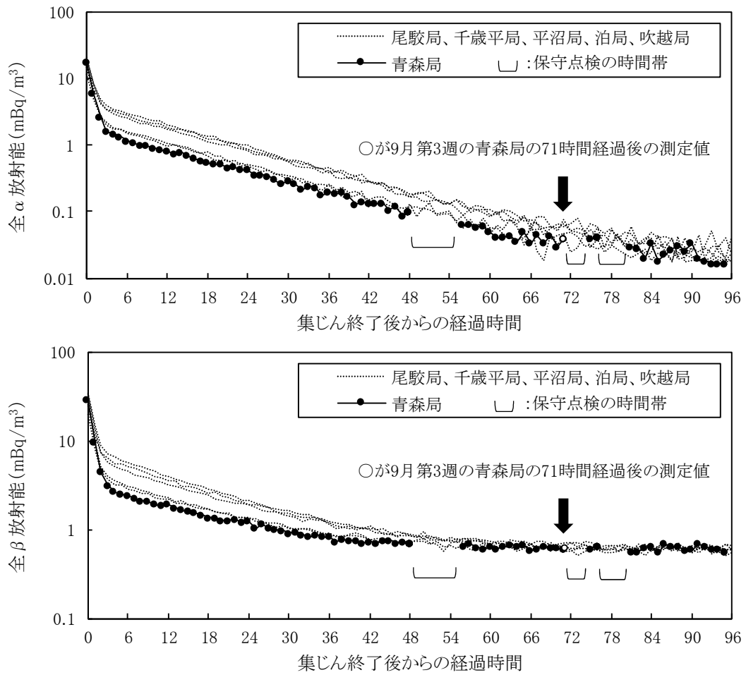
図1 9月第3週の大气浮遊じん中の全 \alpha 及び全 \beta 放射能濃度の推移
