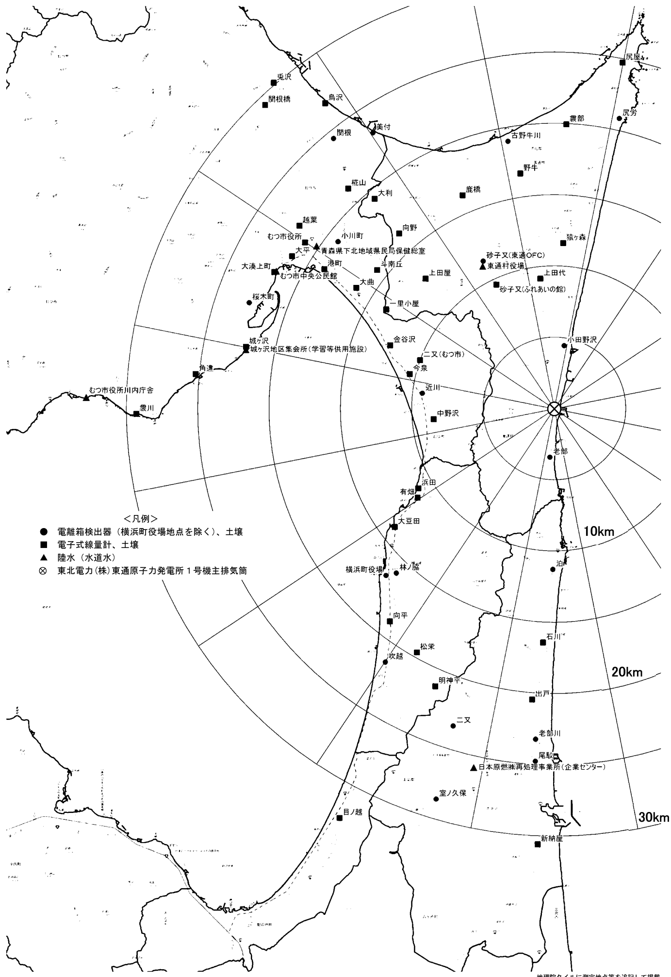
図 2-3 「緊急事態が発生した場合への平常時からの備え」を目的とした調査地点（空間放射線量率、環境試料）
