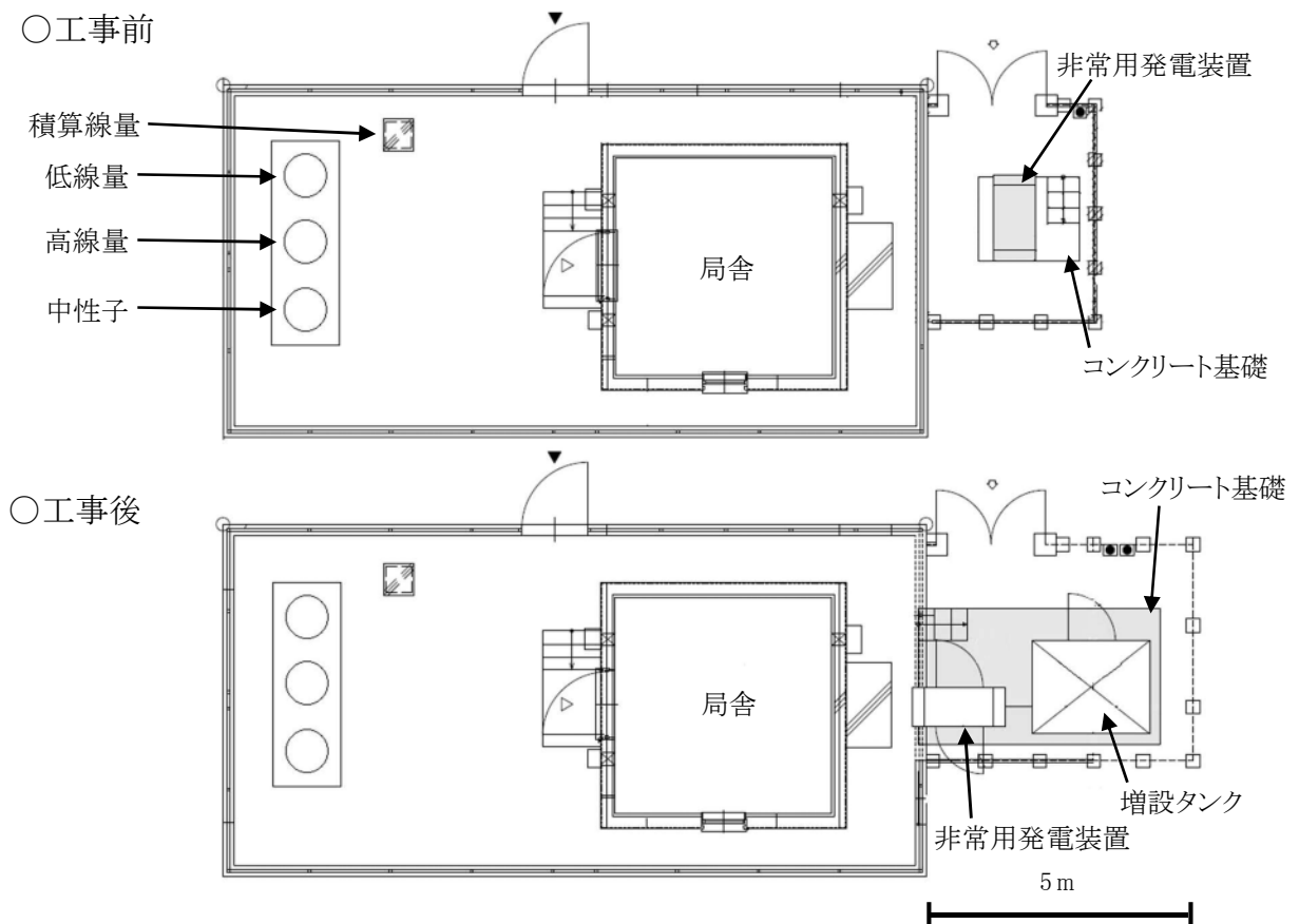
図1 尾駈局の工事概略図
