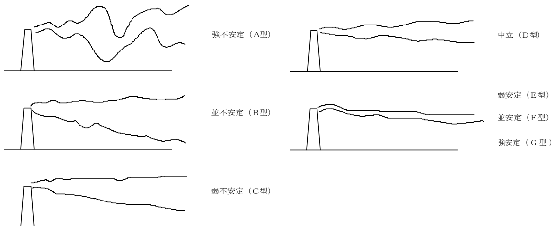
大気安定度と煙の型との模式図
