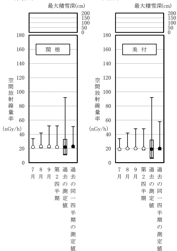
図3-1 モニタリングポストによる空間放射線量率(NaI)測定結果
