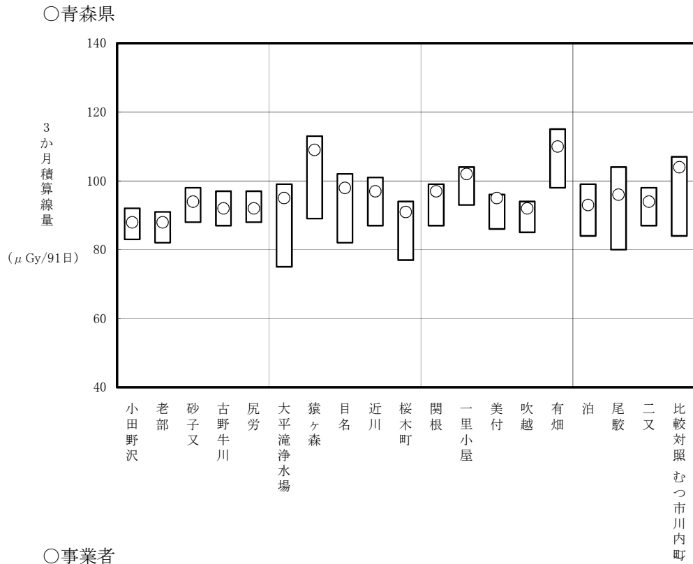
図2-4 RPLDによる積算線量測定結果 (注1)
