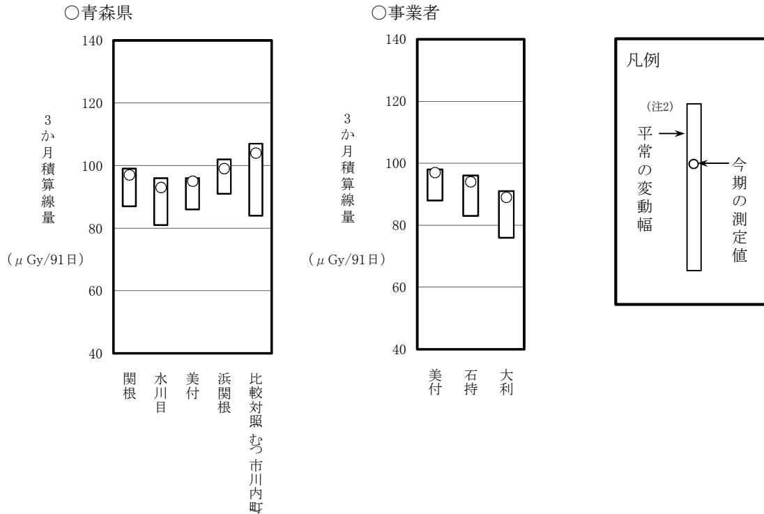
図3-2 RPLDによる積算線量測定結果 (注1)
