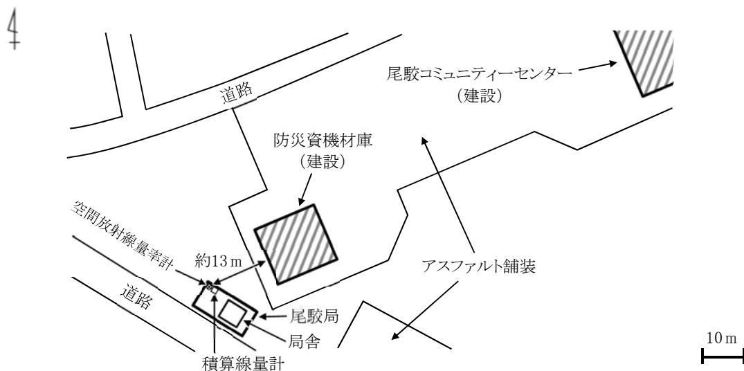
図2 尾駁局周辺の概略図(建設工事関係)
