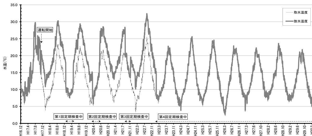
図-1 取放水温度測定結果(日平均)
