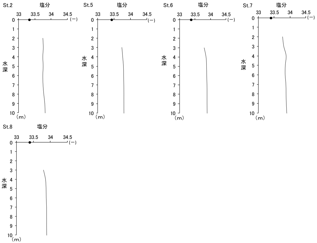
図-2.4 (1.1) 塩分鉛直分布図 (水深10m以浅)
