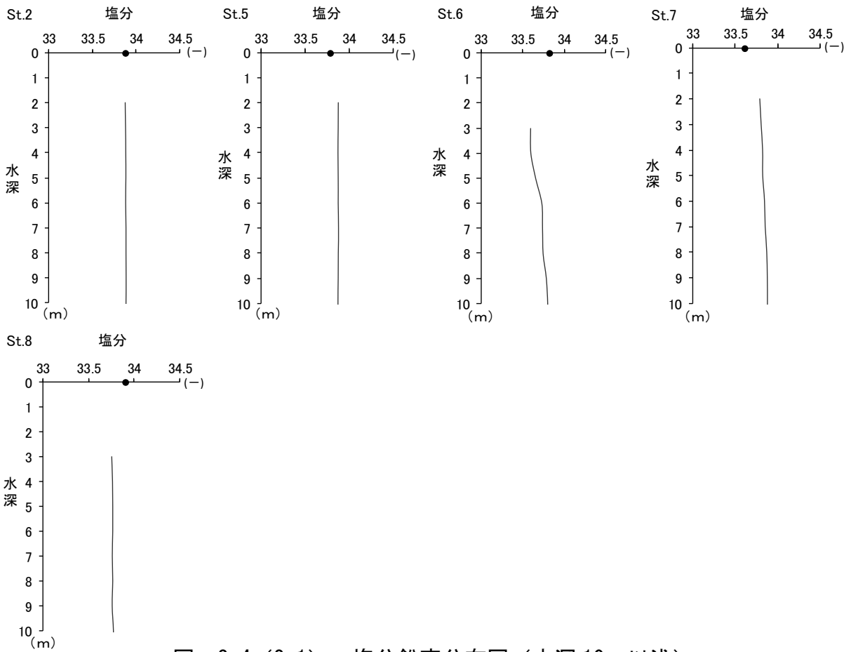
図-2.4 (2.1) 塩分鉛直分布図 (水深 10m 以浅)
