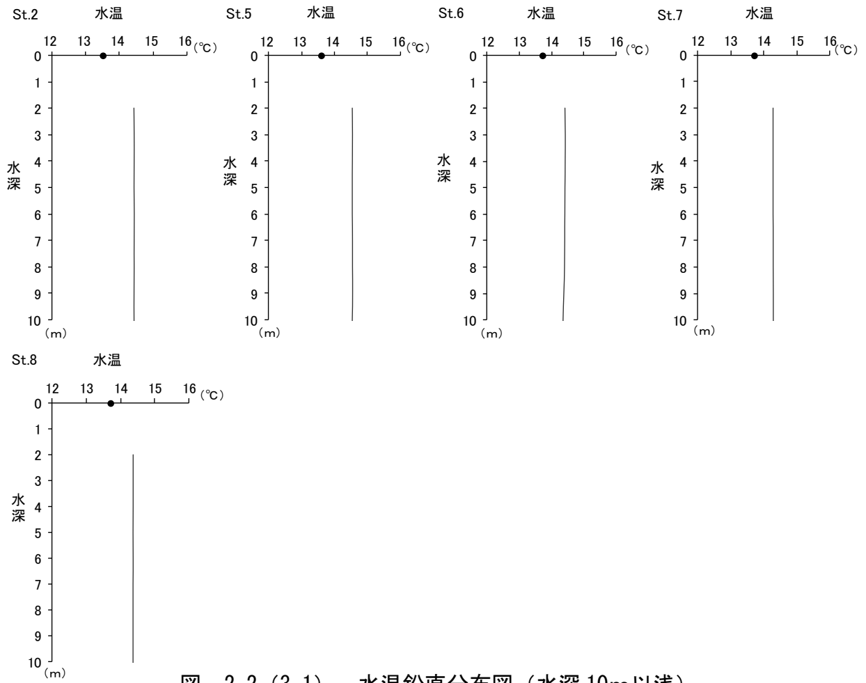
図-2.2 (3.1) 水温鉛直分布図 (水深 10m以浅)
