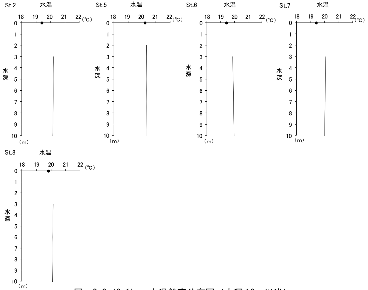
図-2.2 (2.1) 水温鉛直分布図 (水深 10m以浅)
