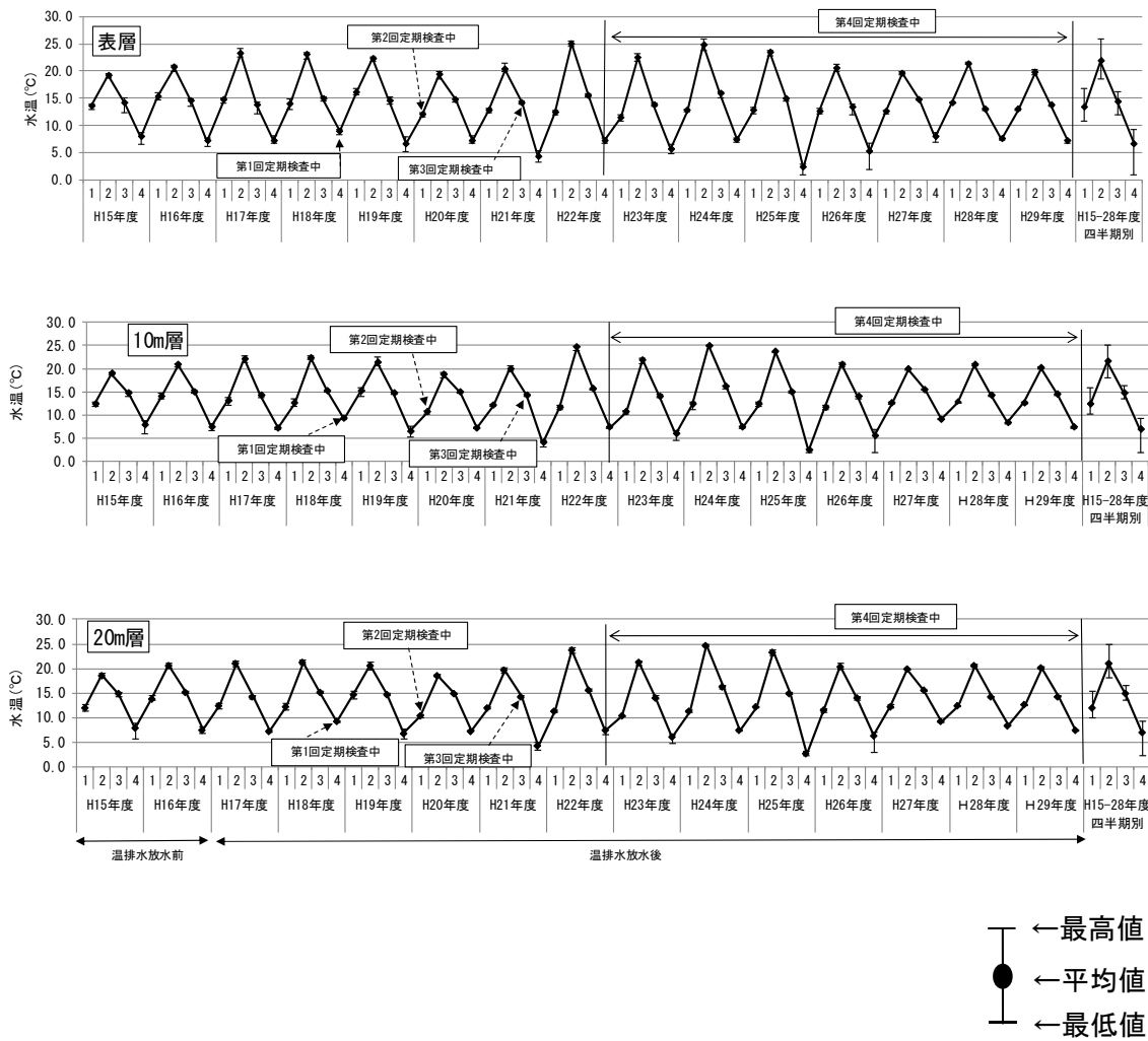
図-1 層別、四半期別の全調査地点平均水温の経時変化
