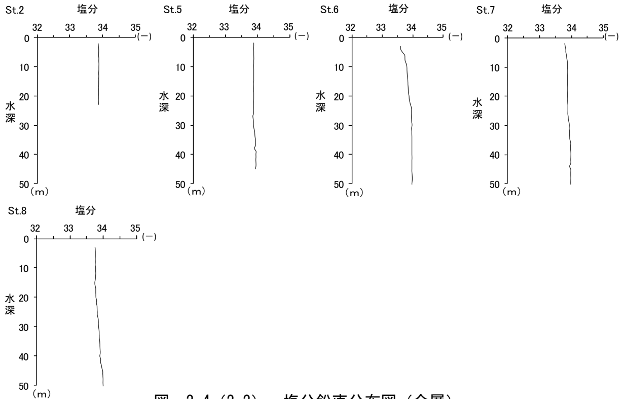
図-2.4 (2.2) 塩分鉛直分布図 (全層)
