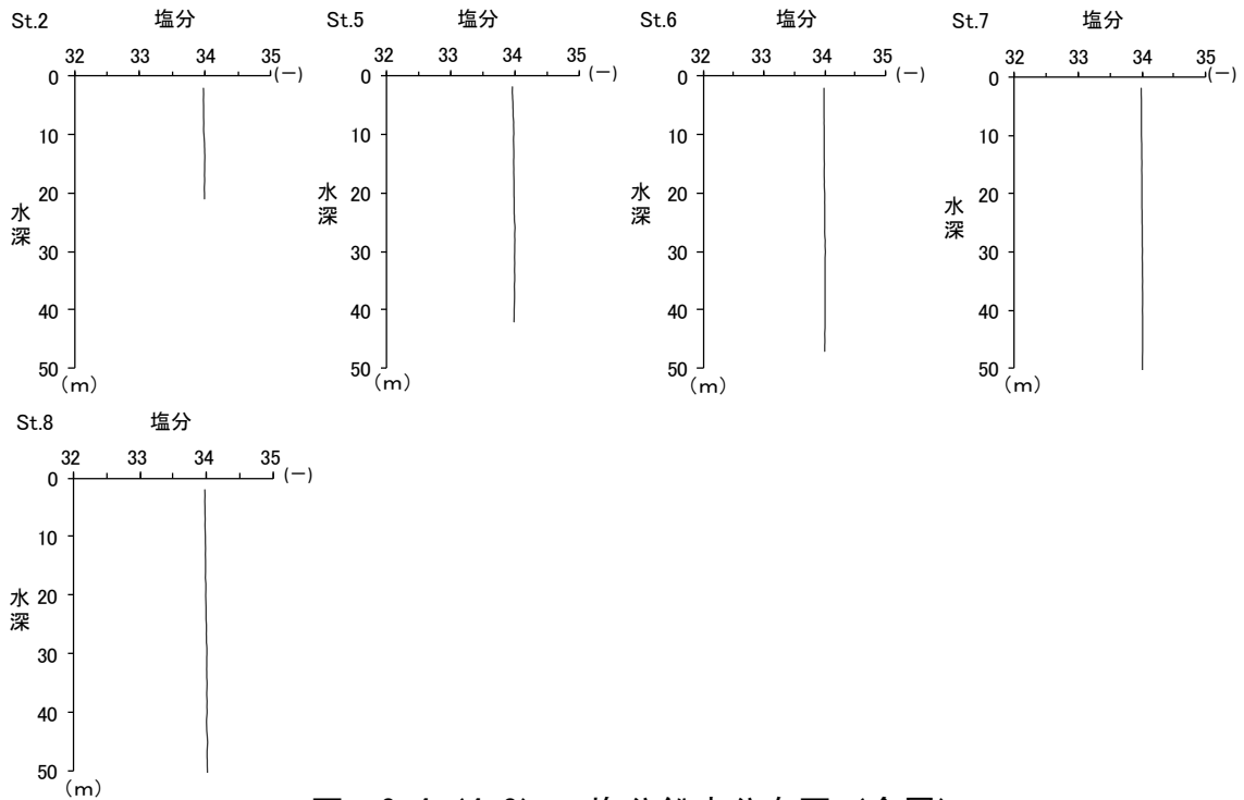
図-2.4 (4.2) 塩分鉛直分布図 (全層)
