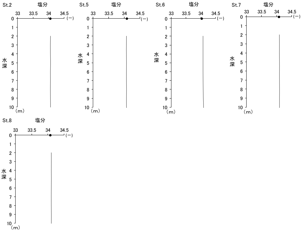
図-2.4 (3.1) 塩分鉛直分布図 (水深 10m以浅)
