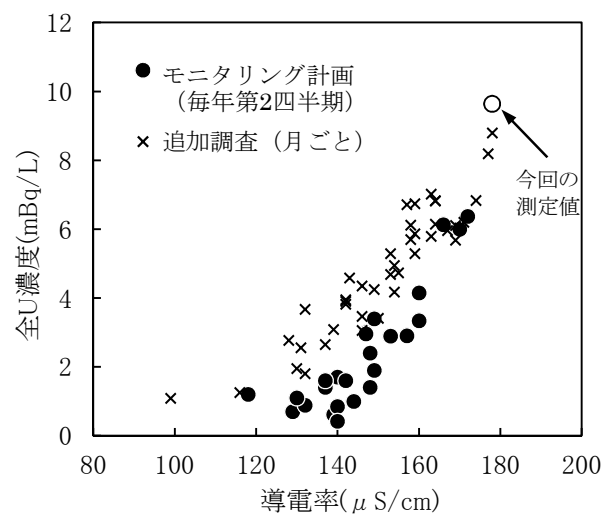
図7 河川水(二又川下流)全ウラン濃度と導電率の関係 (モニタリング計画:平成元年～平成27年、追加調査:平成24年～平成27年)
