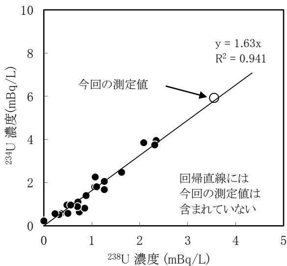
図2 河川水(二又川下流) ^{234}\text{U} 及び ^{238}\text{U} 濃度の相関
