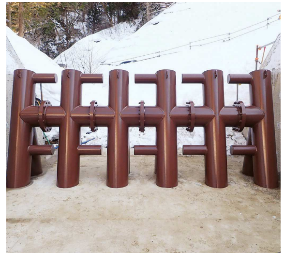
(流木対策) 押付沢総合流域防災砂防事業（六ヶ所村）
