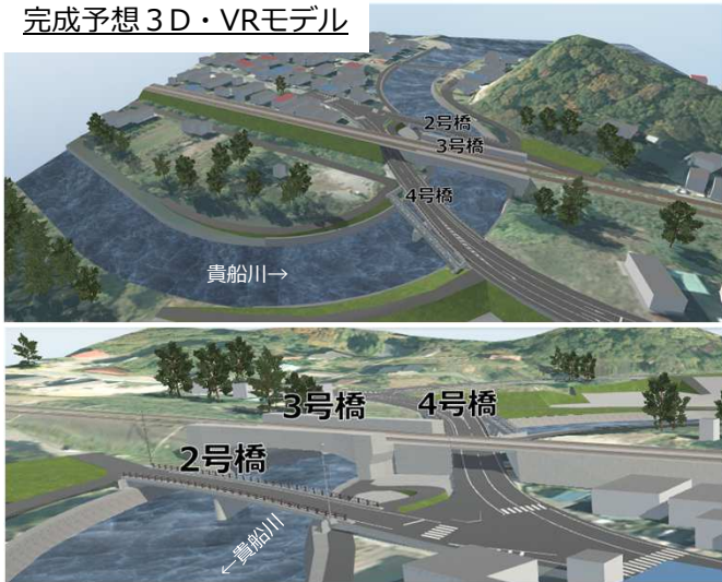
3橋同時施工計画図
