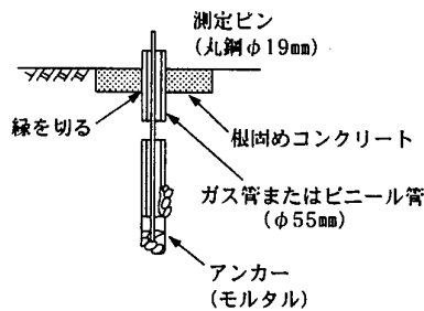
図6-8 地中沈下測定点 of 設置例
