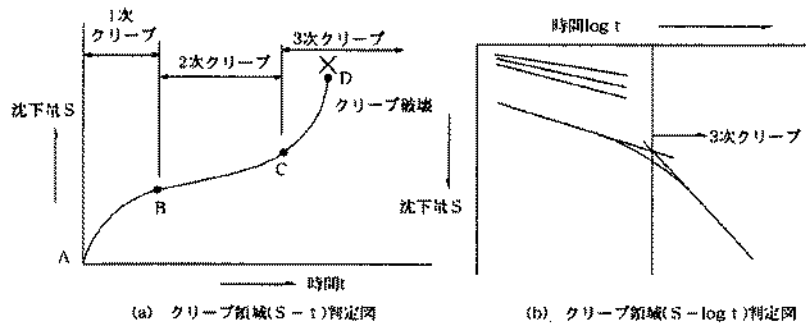
図5-1 天端沈下のクリープ領域判定図
