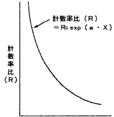
密度あるいは含水量 図-2 計数率比 (R) と密度 及び含水量の関係
