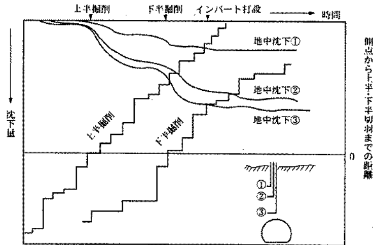
図 6-12 地中沈下量経時変化
