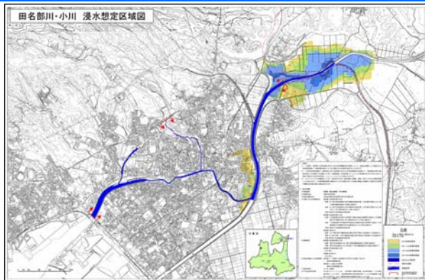
浸水想定区域図（田名部川・小川）
