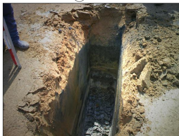
試掘 (a) 完了 (H=2.0m)
