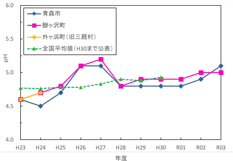
図2 酸性雨経年変化
