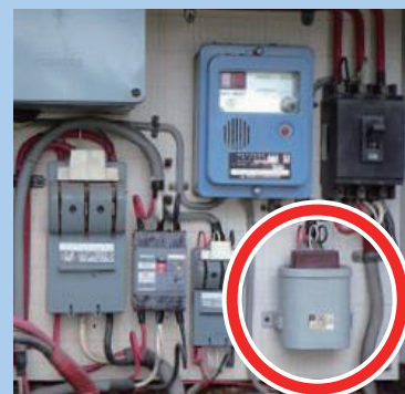
低圧分電盤内の 低圧コンデンサー
