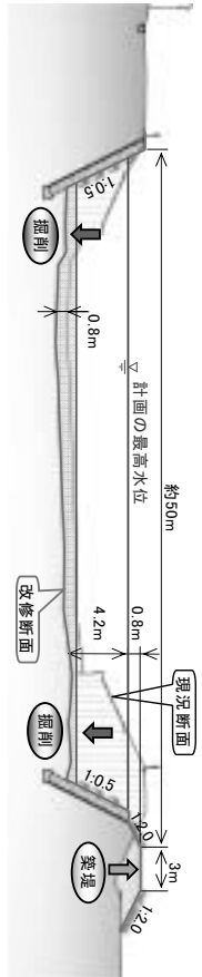
No. 0 (河口) ~ No. 900 (河口から900m)
