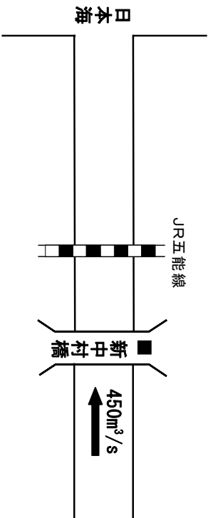
図 2 - 2 整備目標流量配分図
