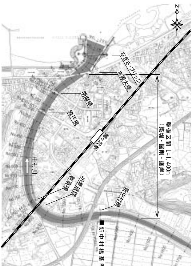
図 3 - 1 中村川河川整備実施位置図
