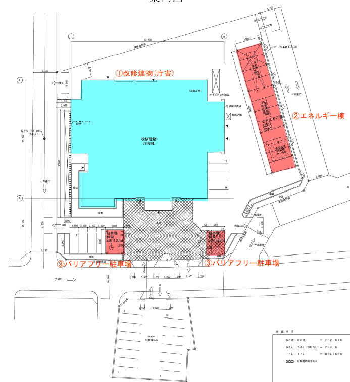
配置図
