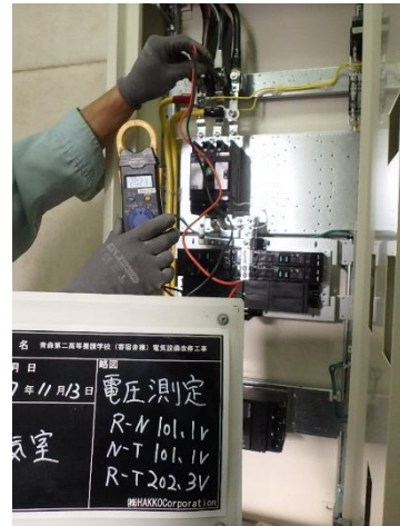
新設電灯分岐盤 試験状況
