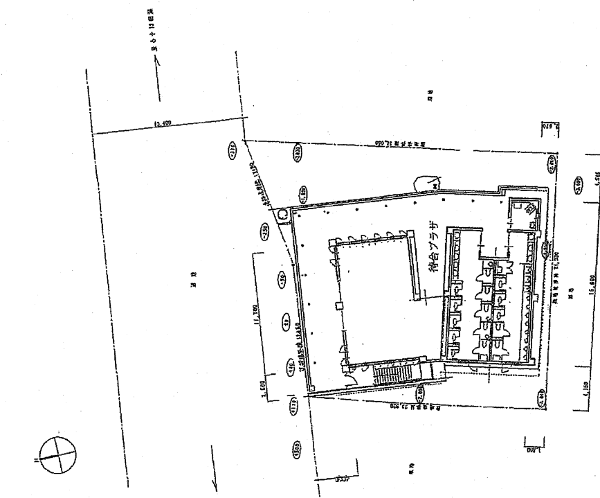
【石ヶ戸休憩所 配置図】
