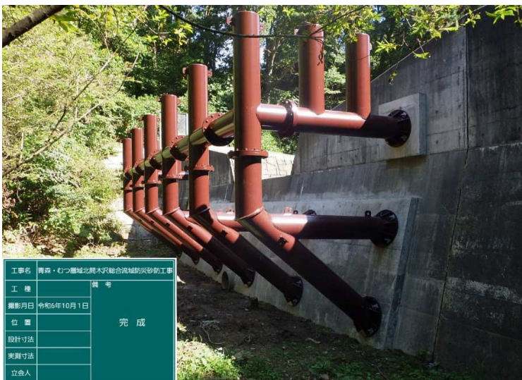
■青森・むつ圏域北間木沢総合流域防災砂防工事_平内町 完成検査：令和6年10月16日
