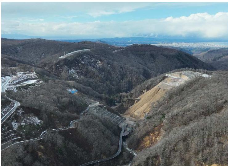
■駒込ダム本体建設工事_青森市(上流より) 出来形検査：令和7年2月26日
