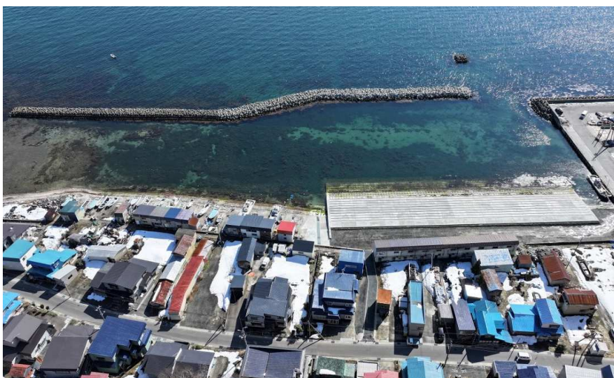
■小湊港地方創生推進船揚場（改良）工事_平内町 完成検査：令和7年3月25日
