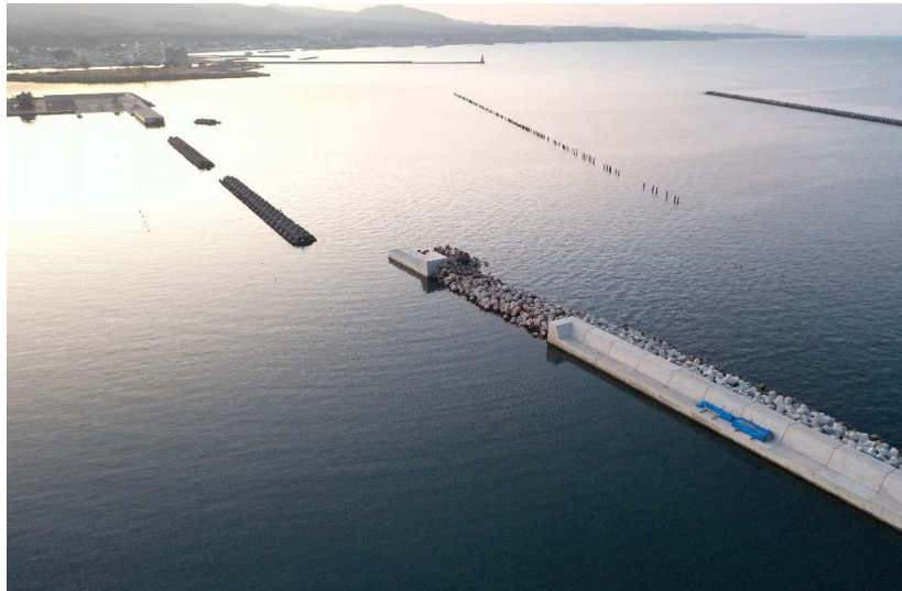
■野辺地地区水産生産基盤整備工事_野辺地町 完成検査：令和6年12月10日
