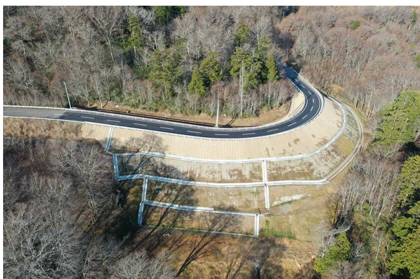
■国道338号道路災害復旧工事_むつ市川内町 完成検査：令和6年12月23日
