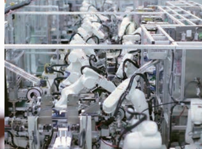
トナーカートリッジの自動生産ラインの様子
