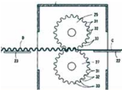
波形ボードの加工装置
