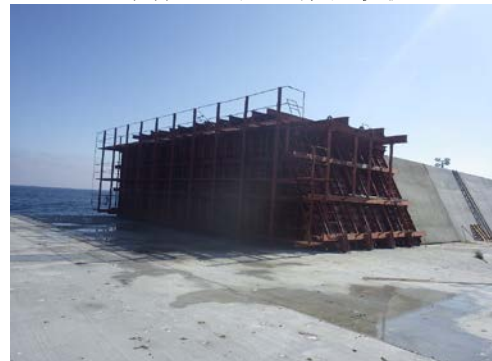
上部工：上部コンクリート打設状況
