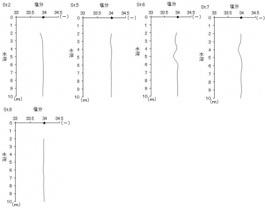
図-2.4 (1.1) 塩分鉛直分布図 (水深10m以浅)
