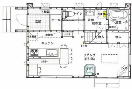
1階平面図 1/100
