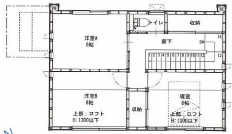
2階平面図 1/100
