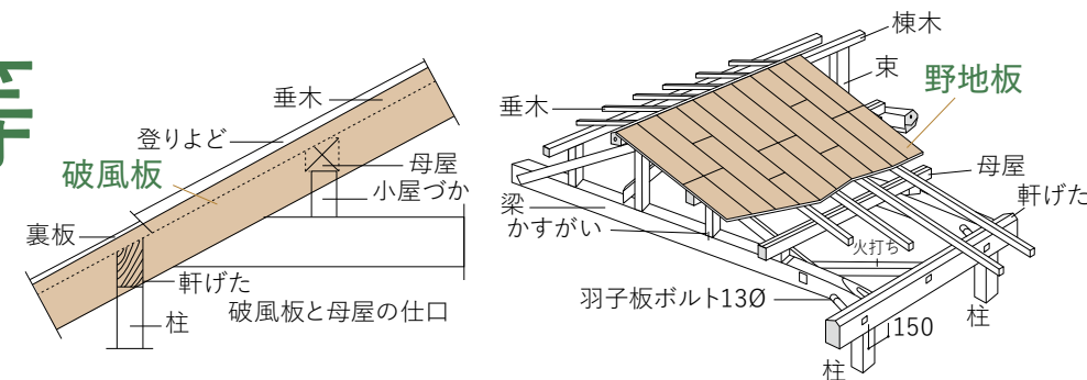
野地板
