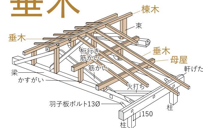
スギ 垂木
