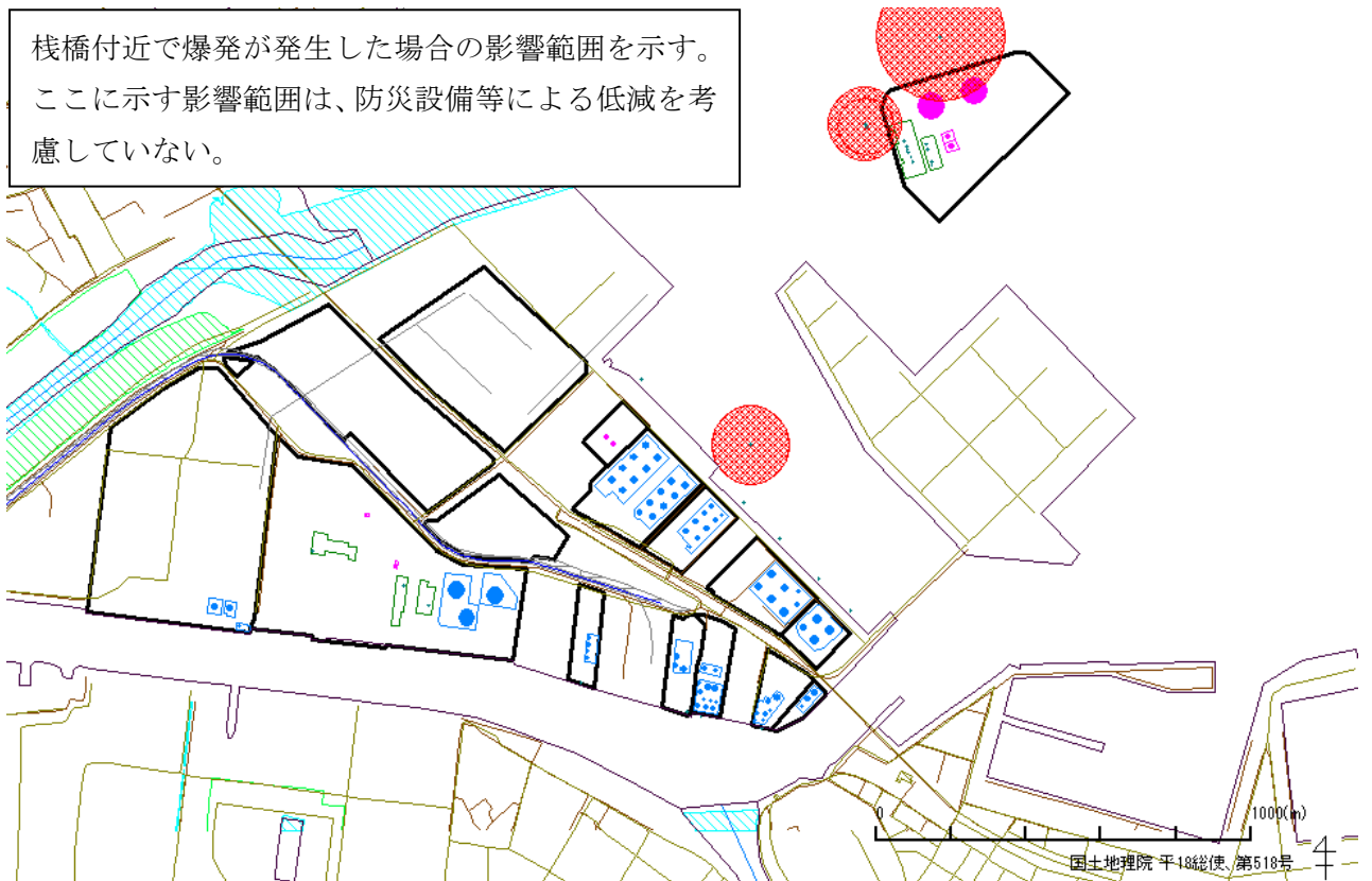
図 4.3.7 八戸地区 可燃性ガスの大規模流出による爆発
