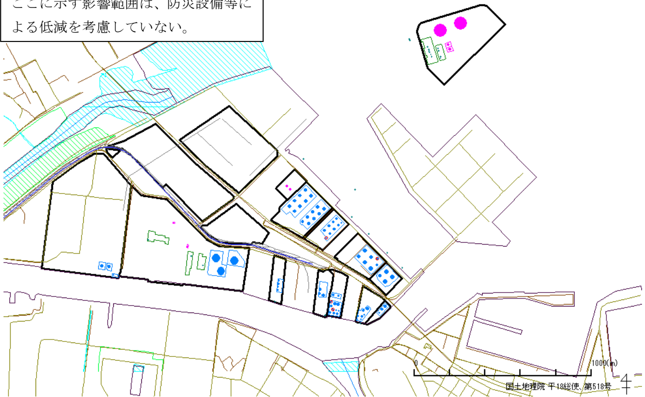
図 1.3.3 八戸地区 危険物タンクのタンク火災(平常時、発生危険度 A・B レベルの災害)
