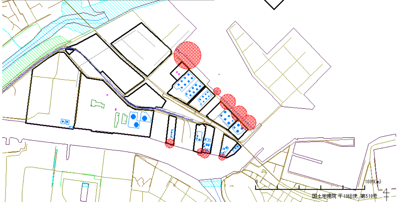
図 4.3.6 八戸地区 タンカー棧橋からの危険物の大規模流出による火災
