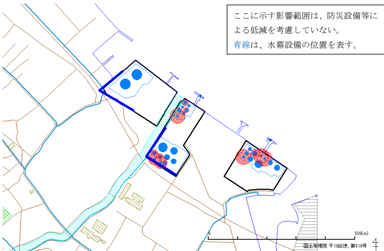
図 1.2.4 青森地区 危険物タンクのタンク火災(平常時、発生危険度 A~C レベルの災害)
