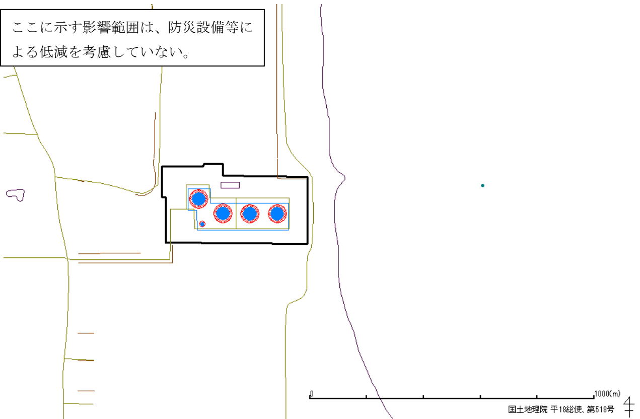
図 1.1.3 むつ小川原地区 危険物タンクのタンク火災(平常時、発生危険度 C レベルの災害) 注) 発生危険度 A・B レベルは該当なし。
