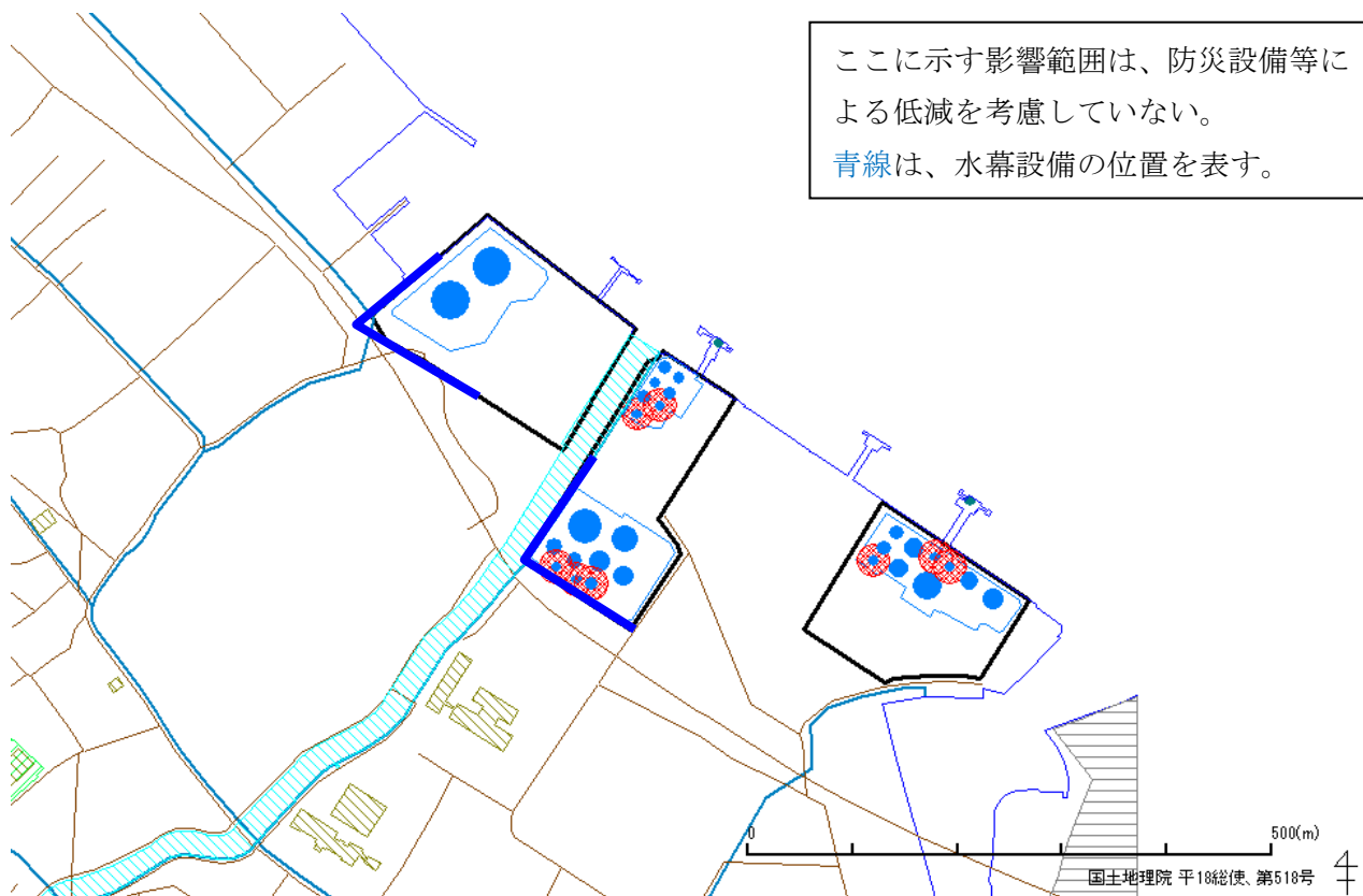
図 2.2.4 青森地区 危険物タンクの流出火災(短周期地震動、発生危険度 C・D レベルの災害)
