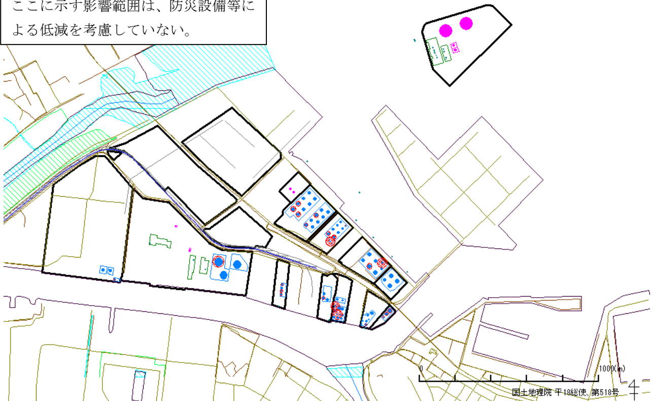
図 1.3.4 八戸地区 危険物タンクのタンク火災(平常時、発生危険度 A～C レベルの災害)
