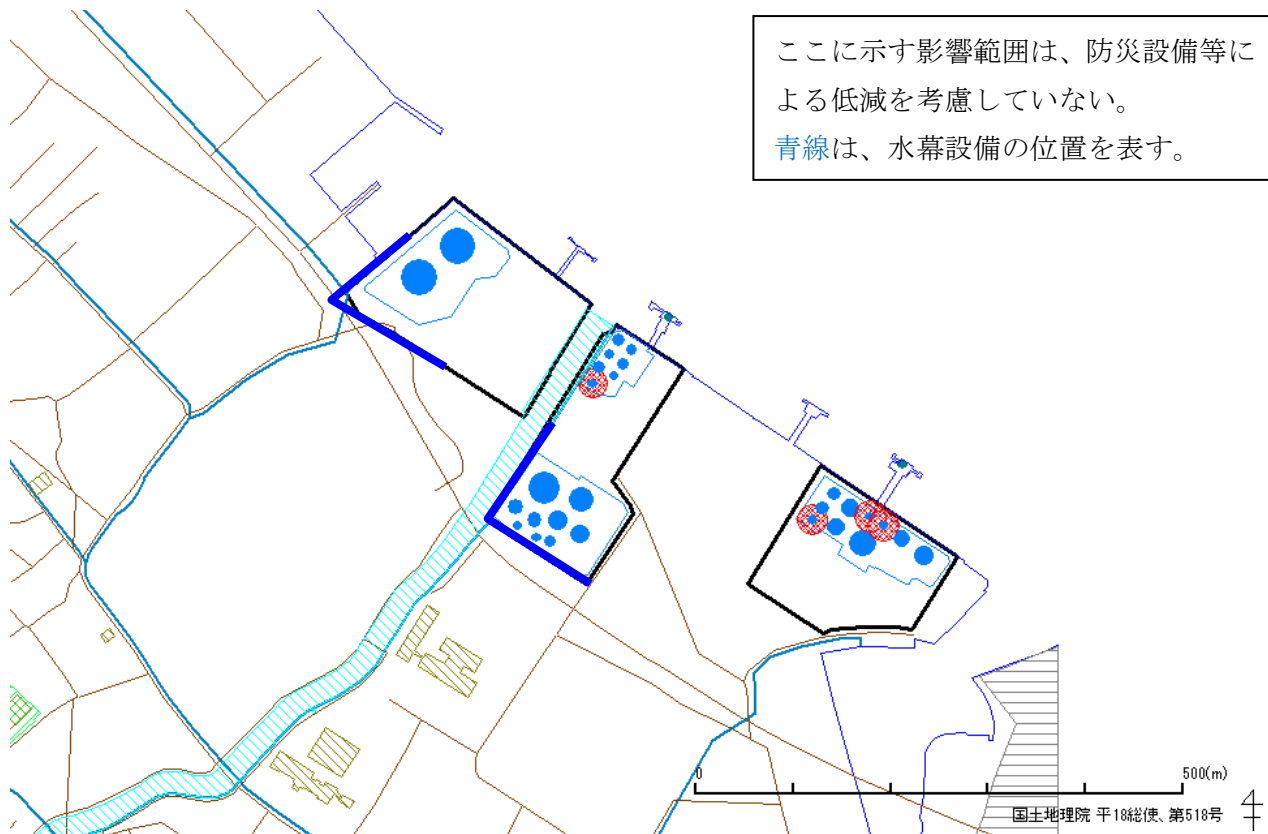
図 2.2.3 青森地区 危険物タンクの流出火災(短周期地震動、発生危険度 C レベルの災害)
