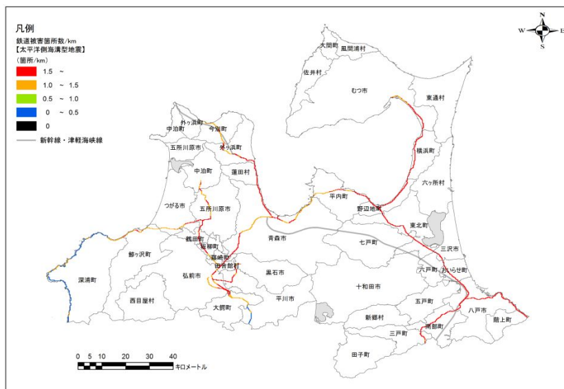
図 5.6.6 鉄道被害
