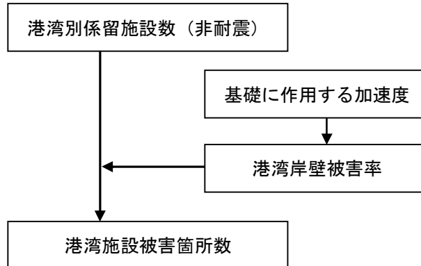
図 5.6.3 港湾被害の予測フロー
