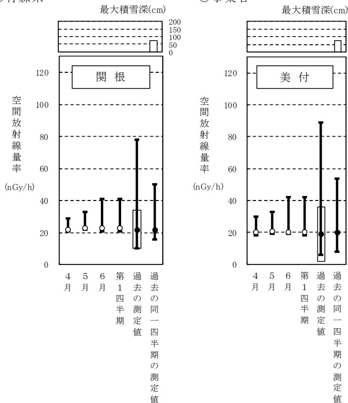
図2-1 モニタリングポストによる空間放射線量率（NaI）測定結果
