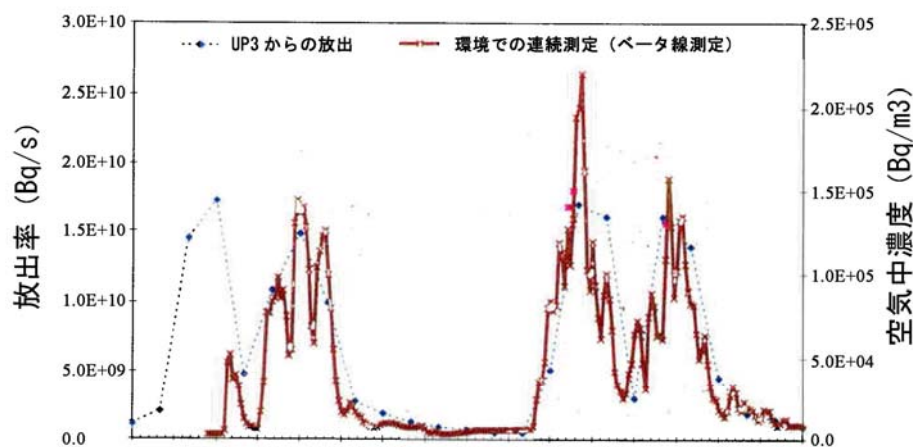
参考図 1. クリプトン-85 放出率および環境での濃度測定値の例 ※1
