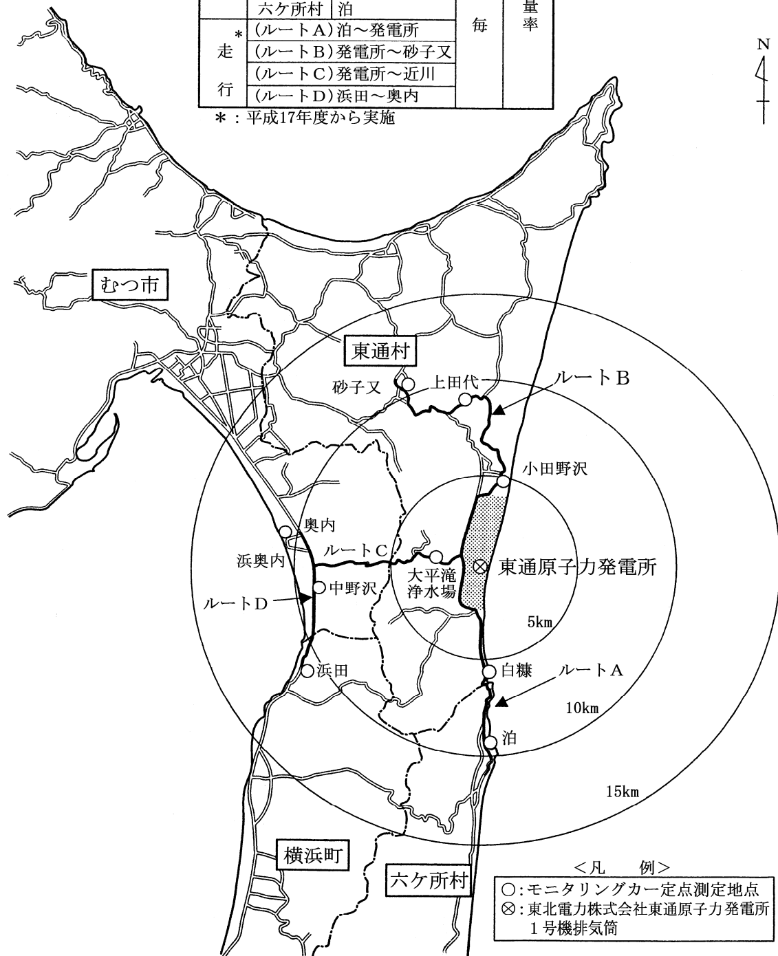
図3 モニタリングカーの定点測定地点及び走行測定ルート
