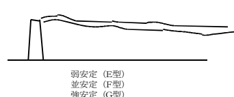
大気安定度と煙の型との模式
