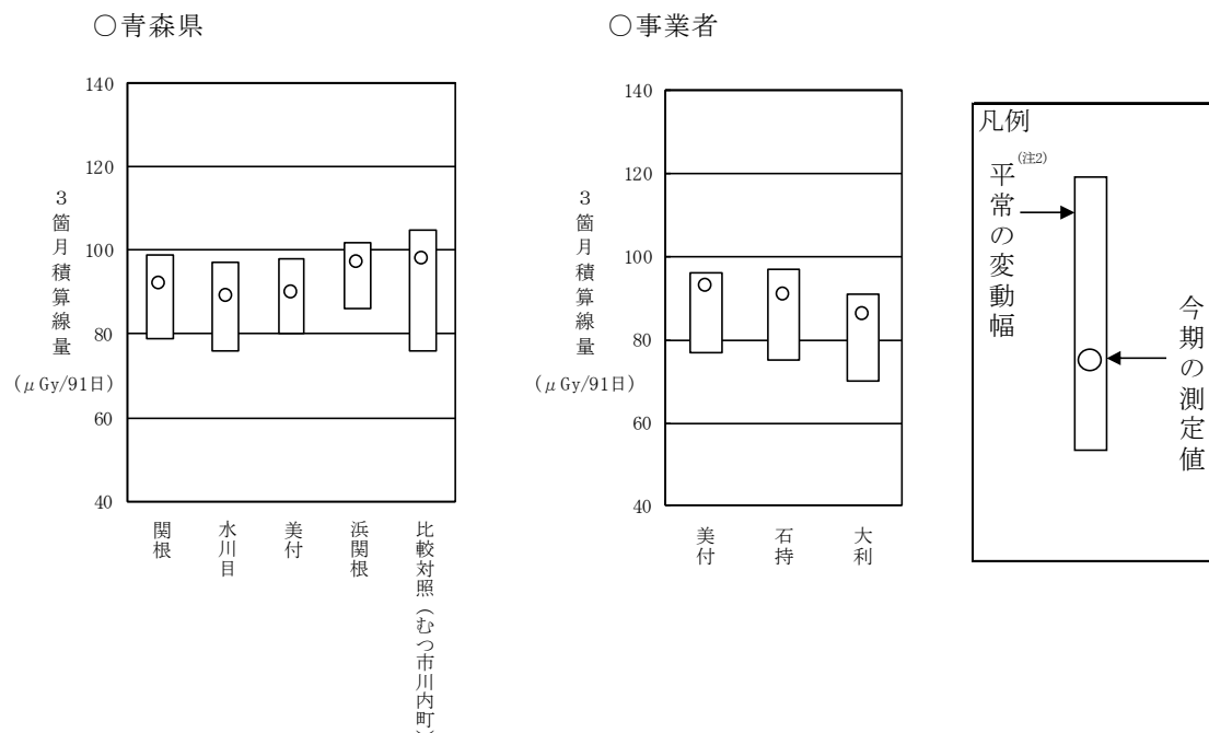
図 2-2 RPLDによる積算線量測定結果 (注1)
