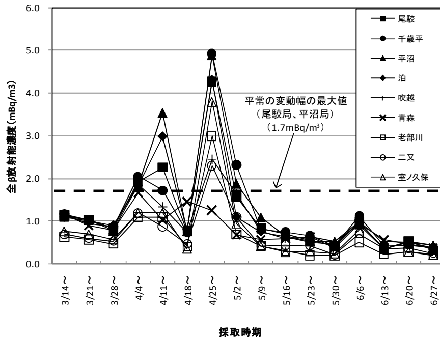
図1 大気浮遊じん中の全 \beta 放射能濃度の推移
