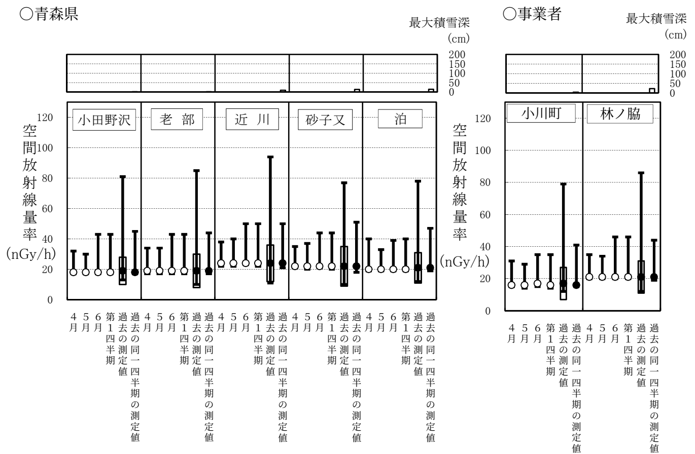
図2-1 モニタリングステーション及びモニタリングポストによる 空間放射線量率（Na I）測定結果
