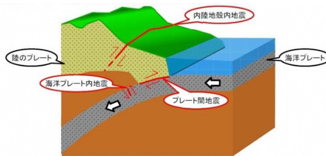
地震発生様式の模式図
