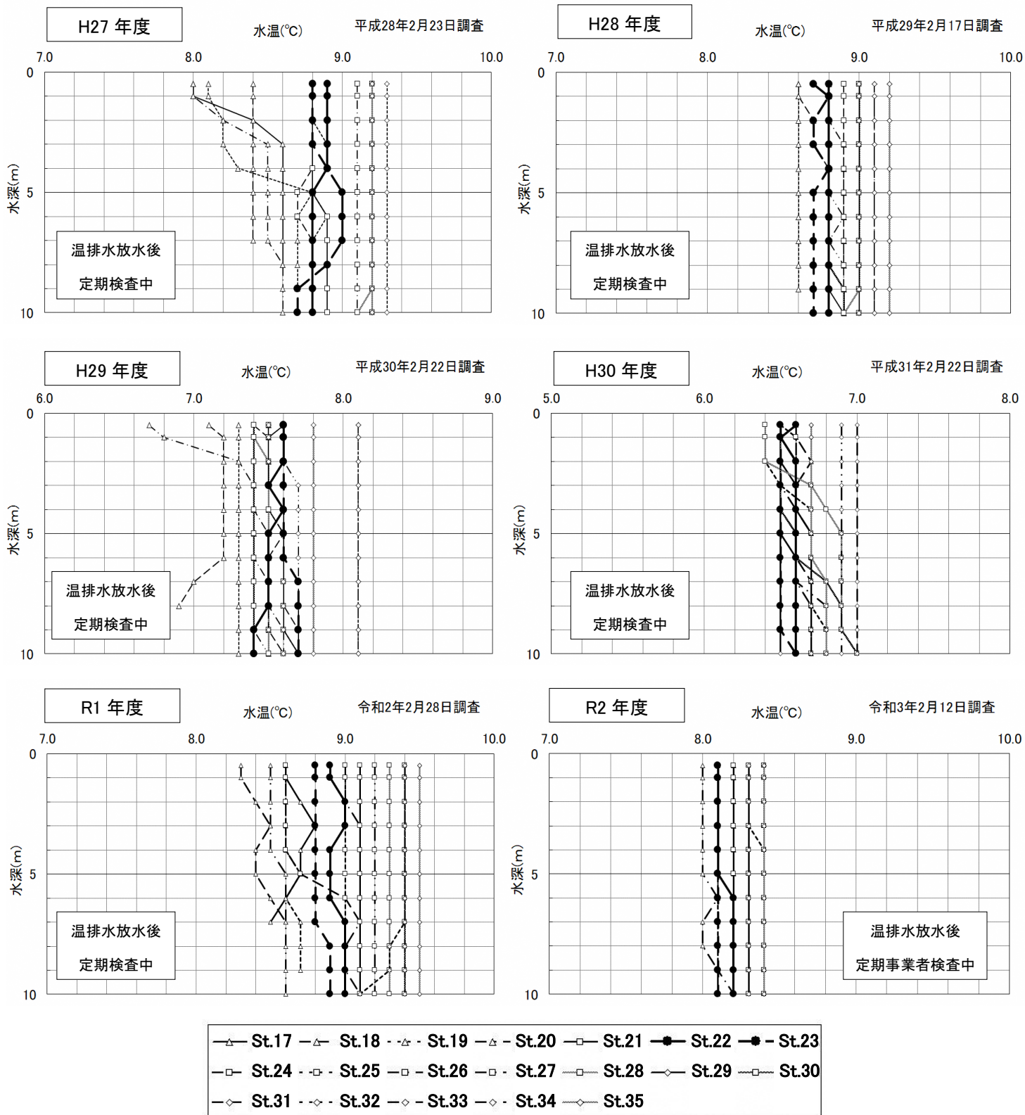
図一3.4(3) 第4四半期水温鉛直分布
