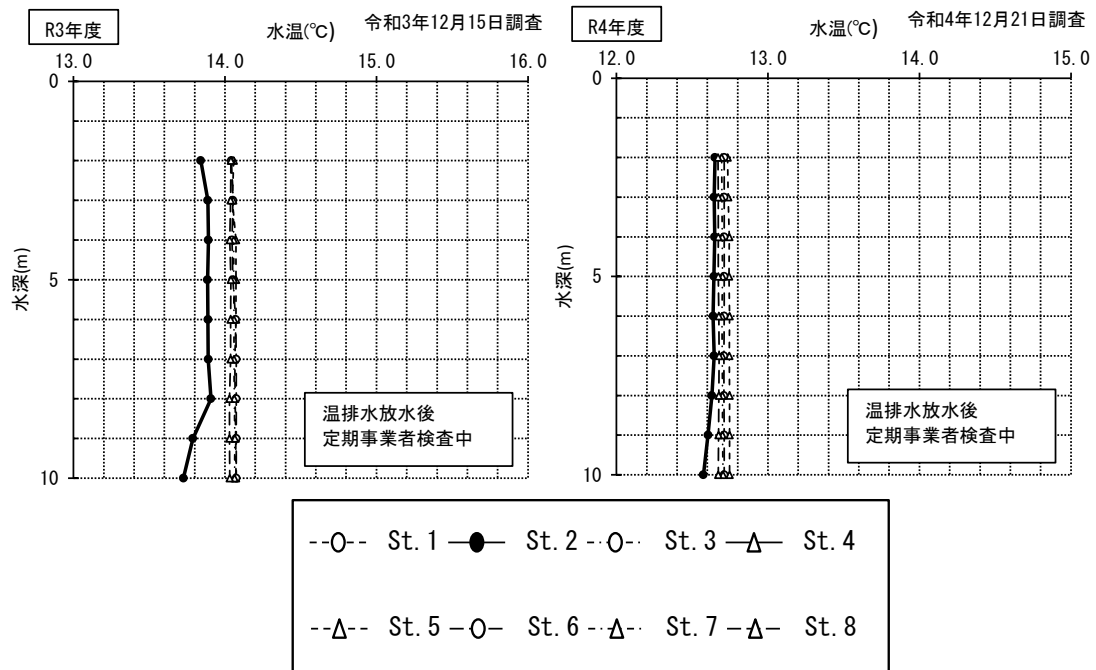
図-2.3 (4) 第3四半期水温鉛直分布
