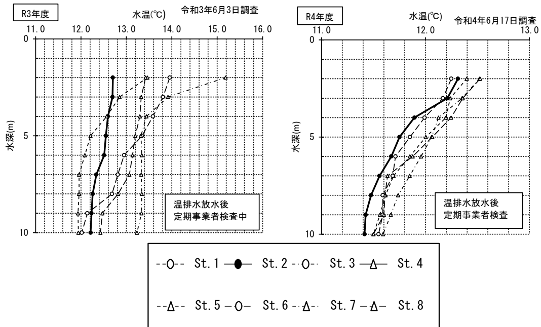
図-2.1 (4) 第1四半期水温鉛直分布
