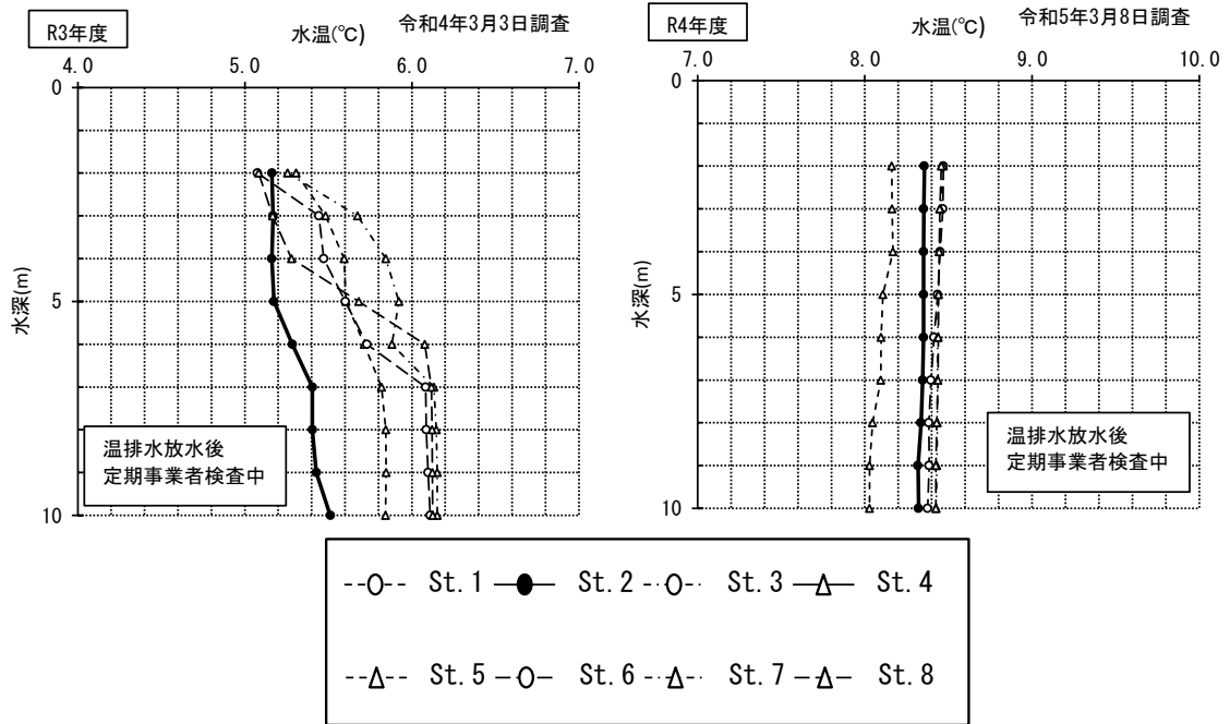
図-2.4 (4) 第4四半期水温鉛直分布
