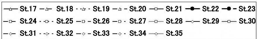
図-3.4(4) 第4四半期水温鉛直分布
