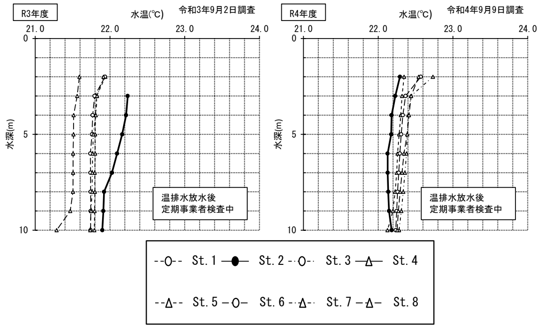
図-2.2 (4) 第2四半期水温鉛直分布
