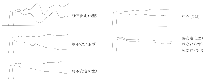
大気安定度と煙の型との模式
