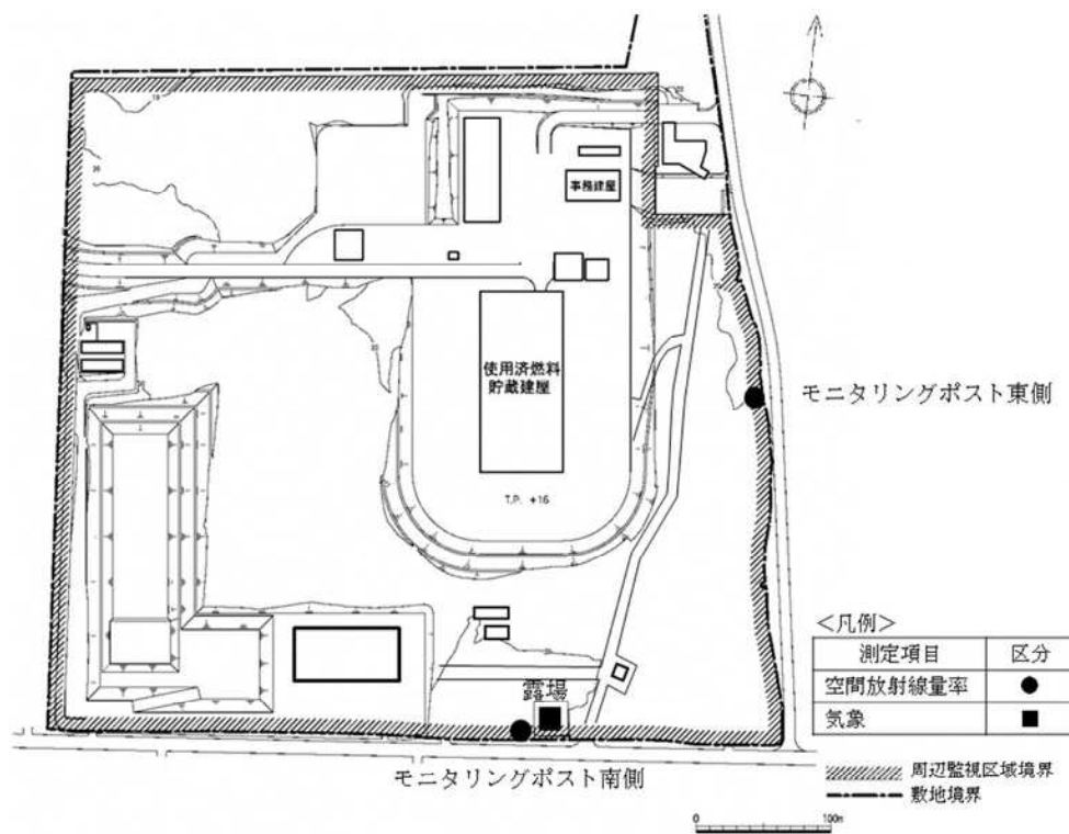
図 使用済燃料貯蔵建屋、モニタリングポスト、気象観測設備配置図
