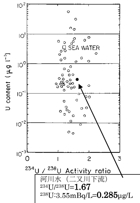
図 3 地表水の ^{234}\text{U}/^{238}\text{U} 放射能比と全ウラン濃度 [1]
