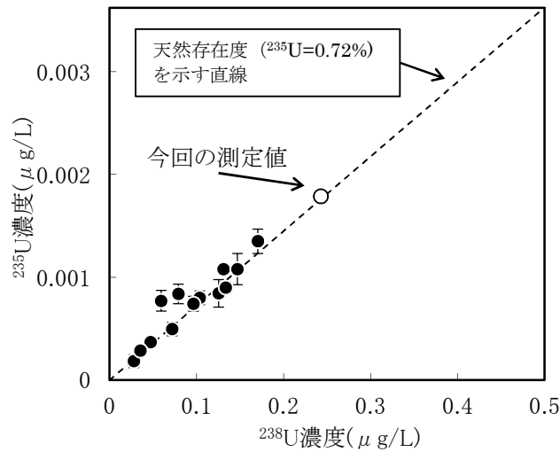
図4 河川水(二又川下流)ICP-MS測定における ^{238}\text{U} と ^{235}\text{U} の相関
