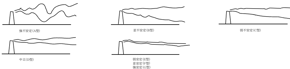
大気安定度と風の型との模式
