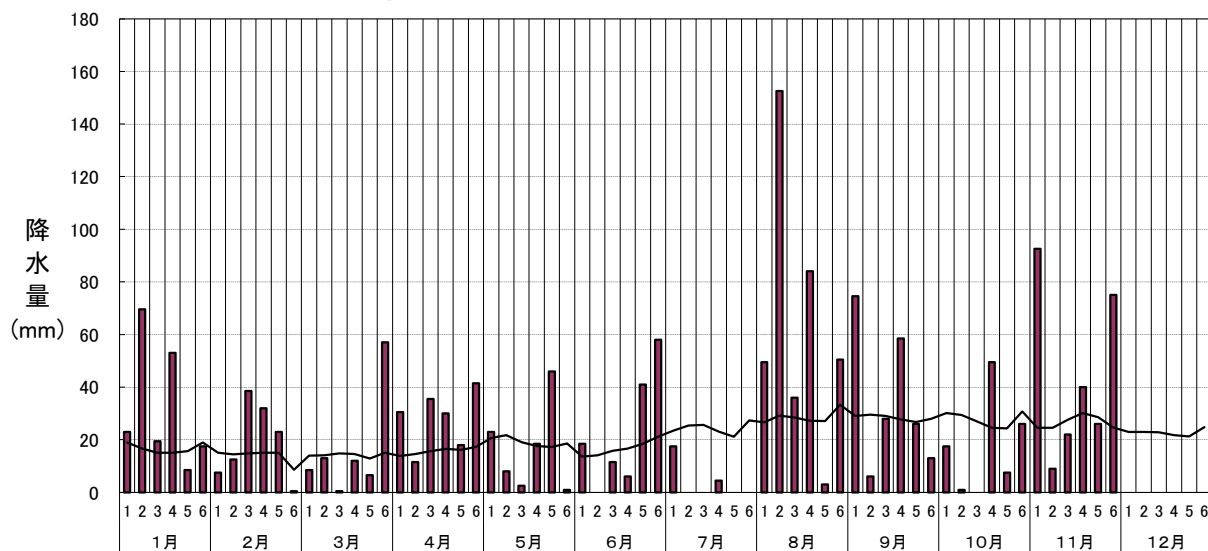
半旬別気象図 降水量(深浦:2025年)
