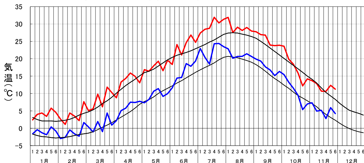
半旬別気象図 最高気温・最低気温(深浦:2025年)
