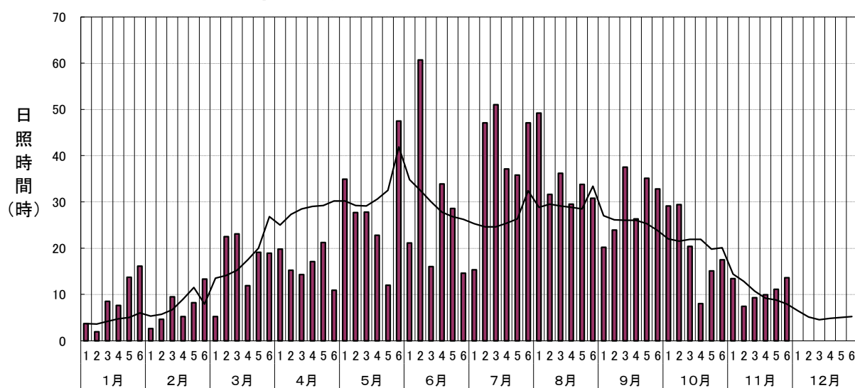
半旬別気象図 日照時間(深浦:2025年)
