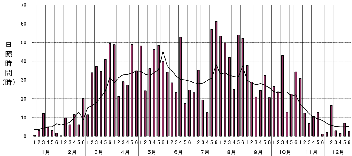
半旬別気象図 日照時間(鱒ヶ沢:2023年)
