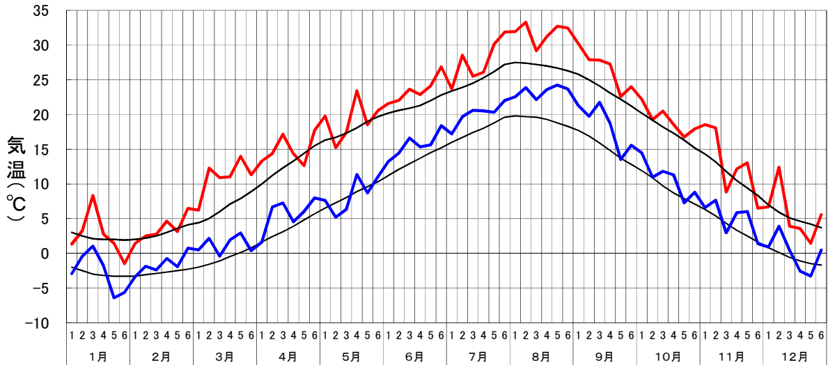
半旬別気象図 最高気温・最低気温(鱒ヶ沢:2023年)
