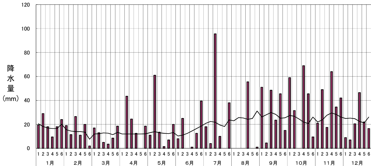
半旬別気象図 降水量(鱒ヶ沢:2023年)
