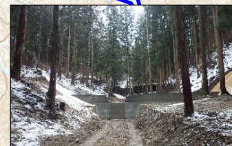
②東田地区で整備中の床固工
