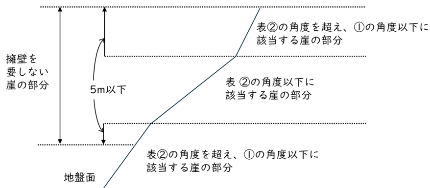
図 2.2.1 擁壁を要しない崖又は崖の部分
