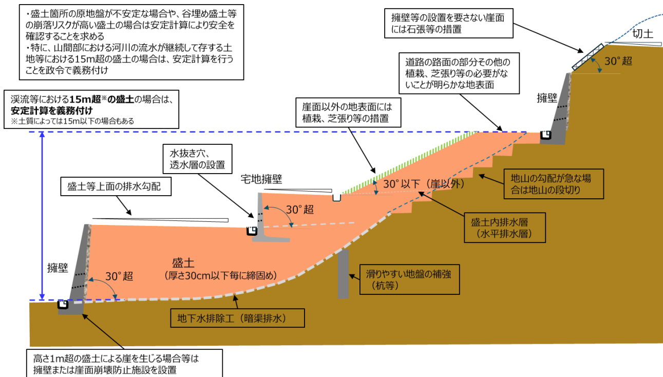
図 1.1.1 土地の形質の変更（盛土・切土）に係る技術的基準の概念図
