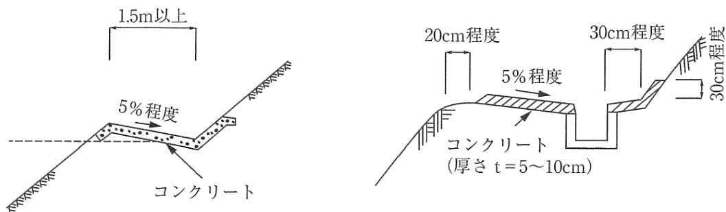
図 7.2.3 小段排水溝
