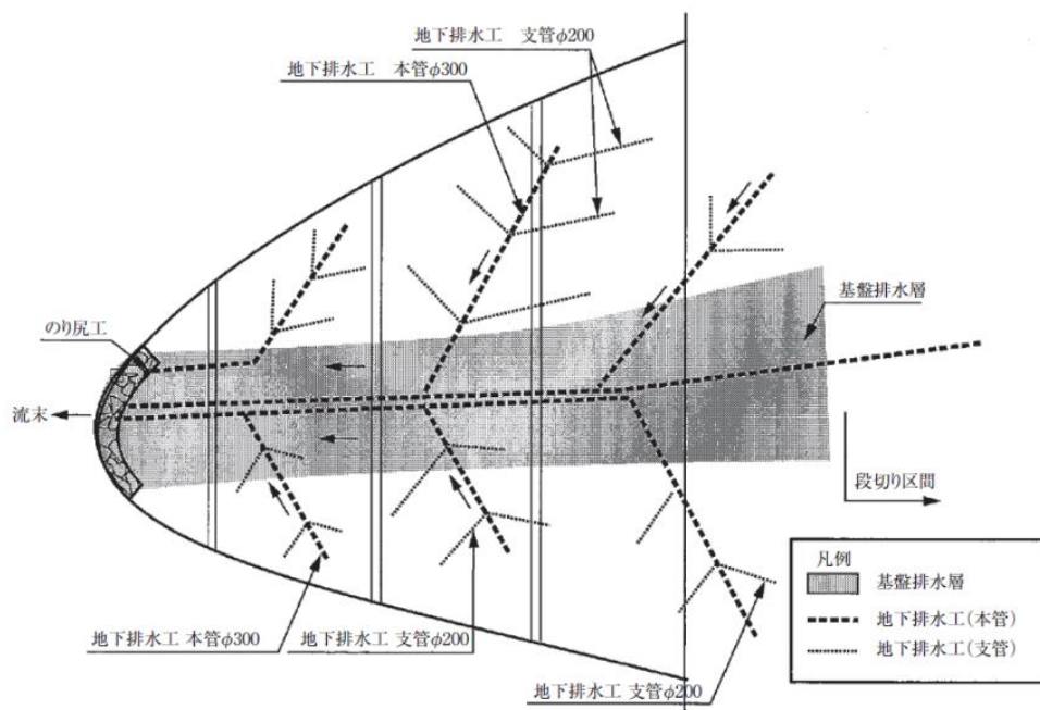
図 7.2.9 渓流等における盛土の暗渠排水工及び基盤排水層の設置例
