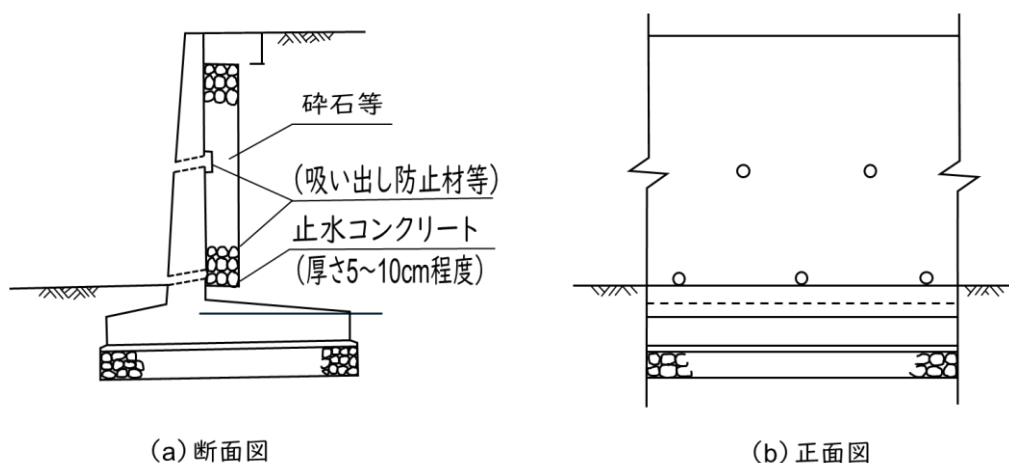
図 3.2.11 水抜き穴の配置図
