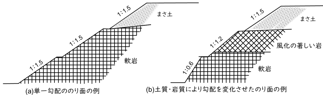
図 2.2.2 地山状態と切土のり面の形状
