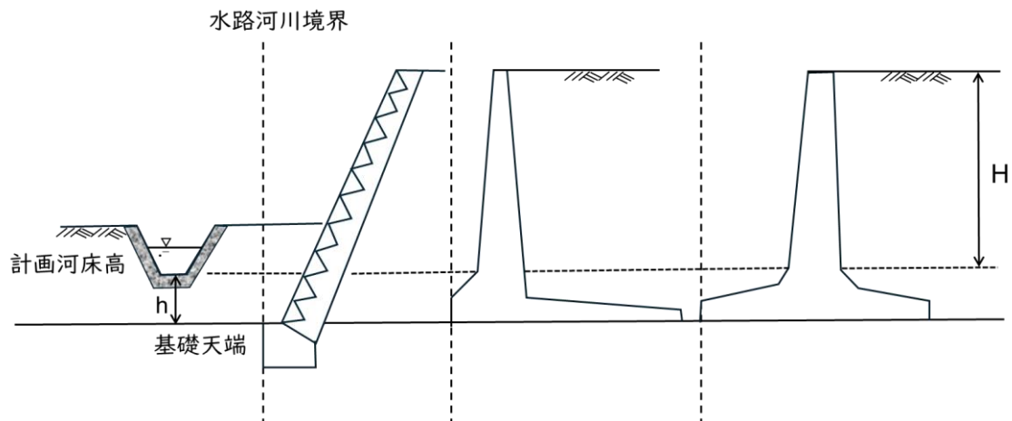
図 3.3.3 根入れの深さ（練積み造擁壁 水路・河川に接する場合）
