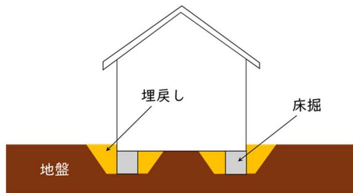
地中埋設物撤去のための床掘り及び埋戻し
