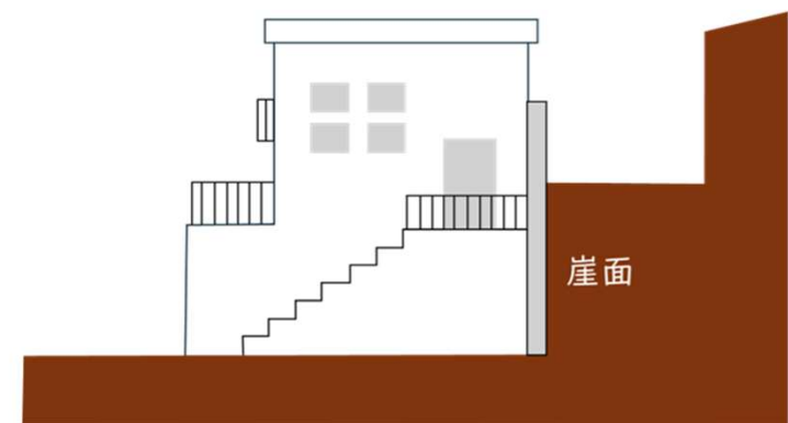
建築物の一部が擁壁を兼ねる場合
