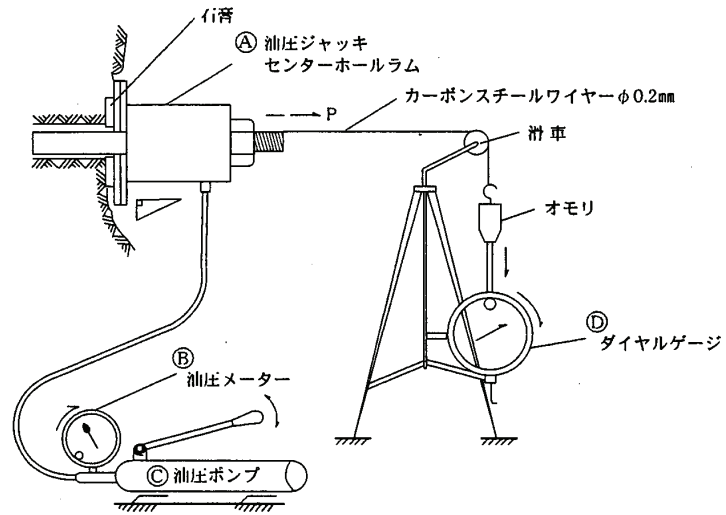
図 4 - 3 引抜試験概要図
