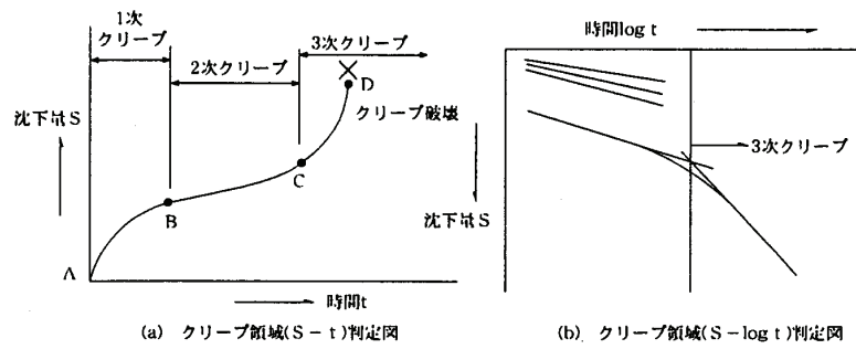
図 5-1 天端沈下のクリープ領域判定図
