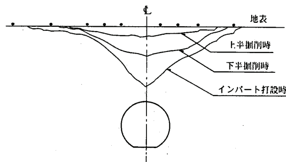
図 6-13 地表沈下分布（横断方向）
