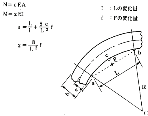
図 6-5 コバリーの図
