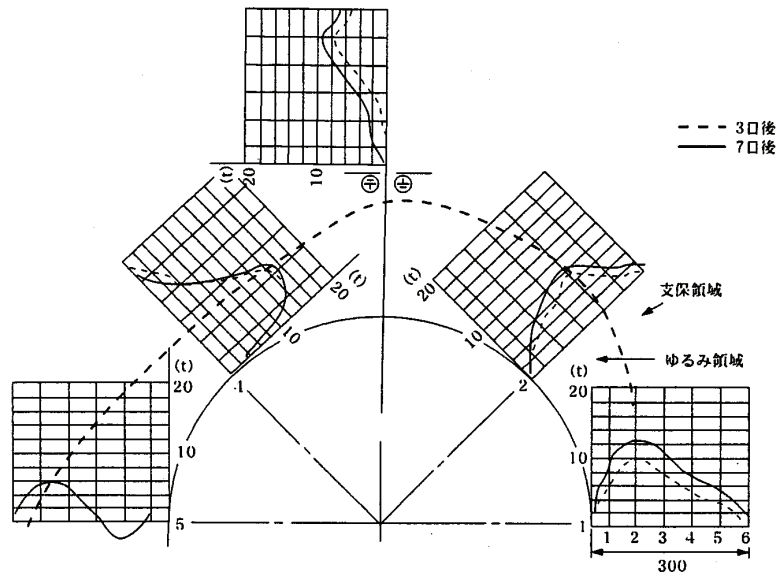
図 6-3 ロックボルトの軸力分布
