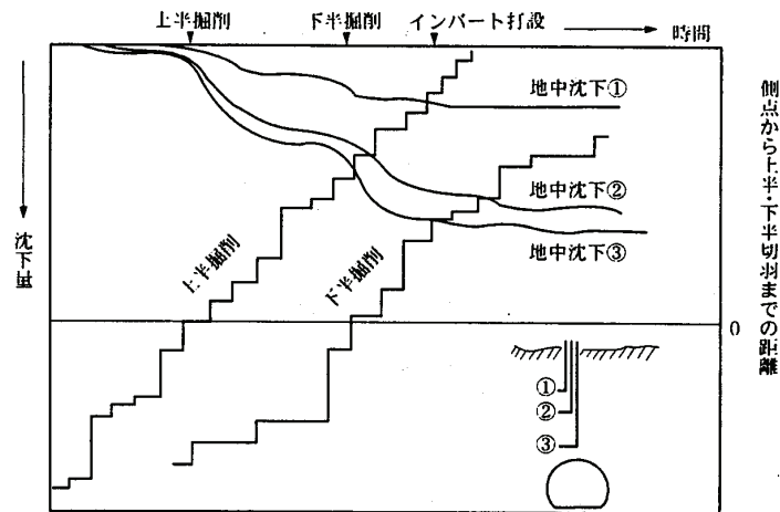
図 6-12 地中沈下量経時変化
