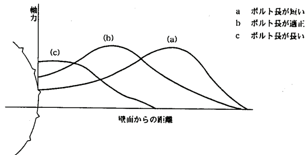
図 6-4 ロックボルトの軸力分布
