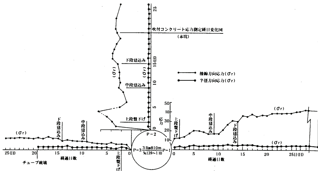
図 6-6 吹付コンクリート応力分布図
