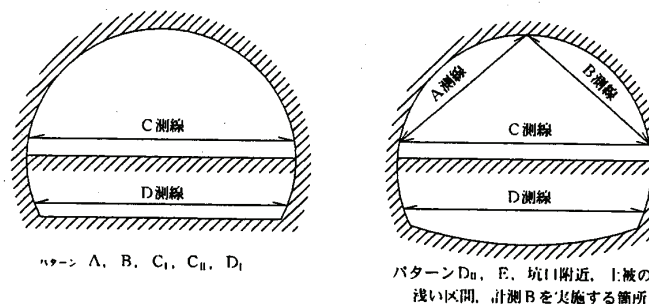
図 5-2 内空変位の測線
