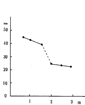
図 6-1 深度～地中変位
