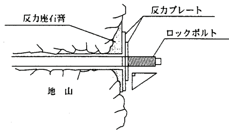
図 4 - 2 反力座の設置
