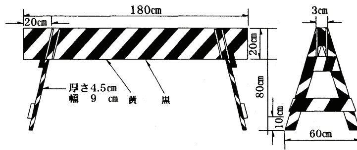
防 止 柵 図1 (一般用その1)
